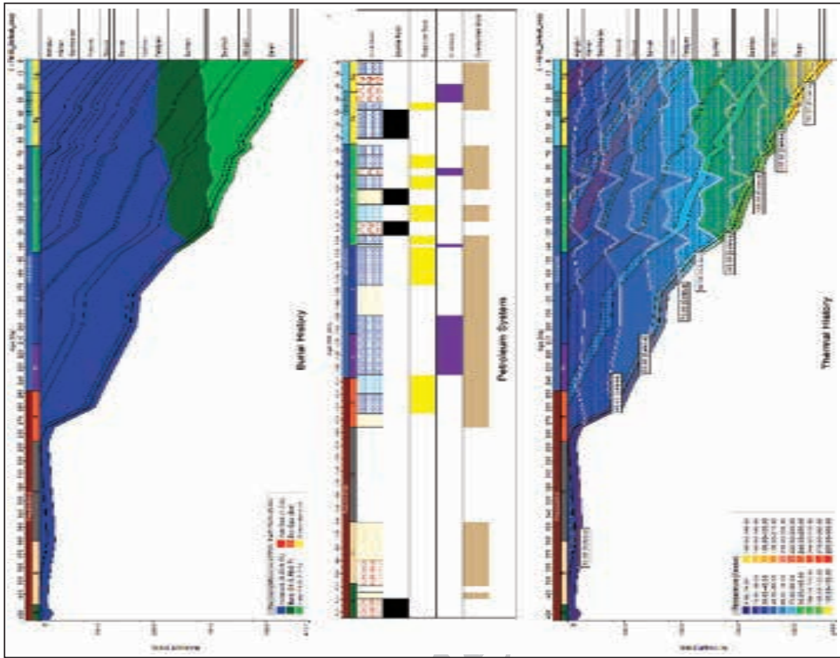
شکل ۶- الف) مدل تاریخچه تدفین و روند پختگی چاه C ب) سیستم های هیدروکربوری این چاه مانند سنگ منشا، سنگ مخزن و سنگ پوشش و ج) تاریخچه گرمایی آن.
