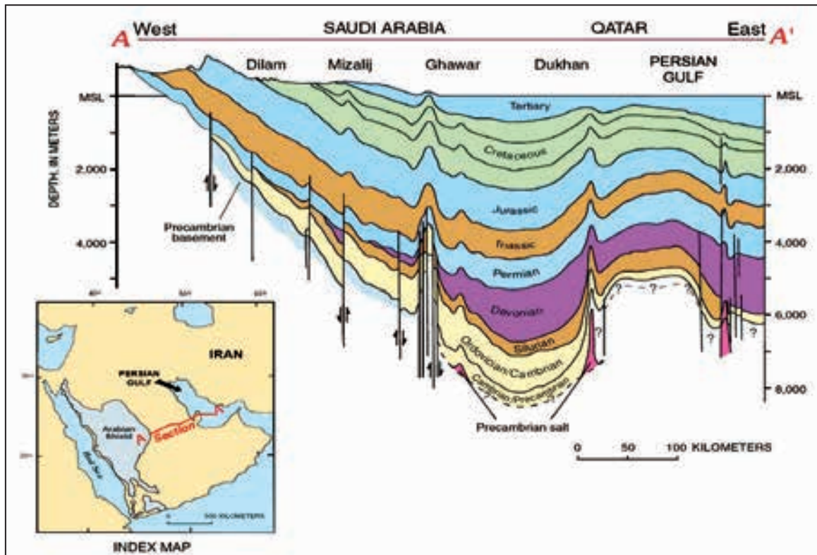
شکل ۲- روند رسوبی پر کامبرین تا عهد حاضر از سمت سپر عربی به سمت حوضه خاوری خلیج فارس. (برگرفته از Al-Sharhan and Narin, 1997 و Konert et al., 2001).
