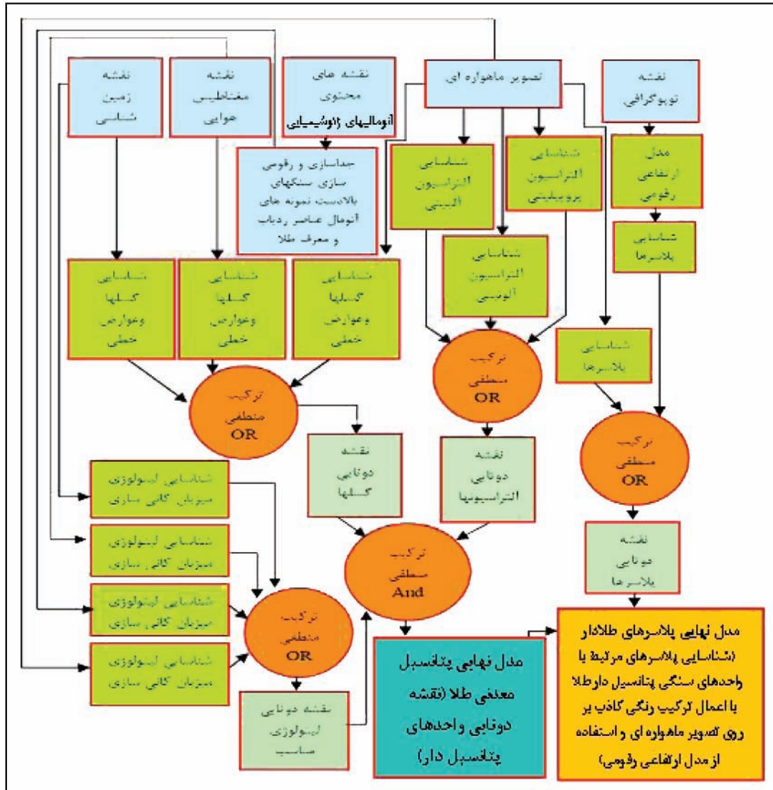
شکل ۳- الگوریتم بهینه تولید مدل پتانسیل معدنی در اکتشاف مقدماتی ذخایر طلا.
