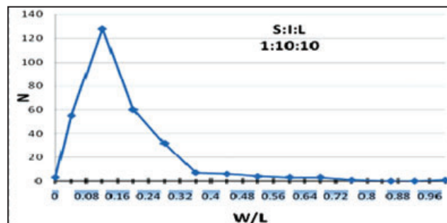
شکل ۱۱- نمودار برآورد ابعاد بلورهای پلاژیو کلاز (محور افقی مقدار عرض میکروولیت های پلاژیو کلاز تقسیم بر طول میکروولیت ها در مقاطع میکروسکوپی و محور عمودی فراوانی بلورها در هر بازه است).
