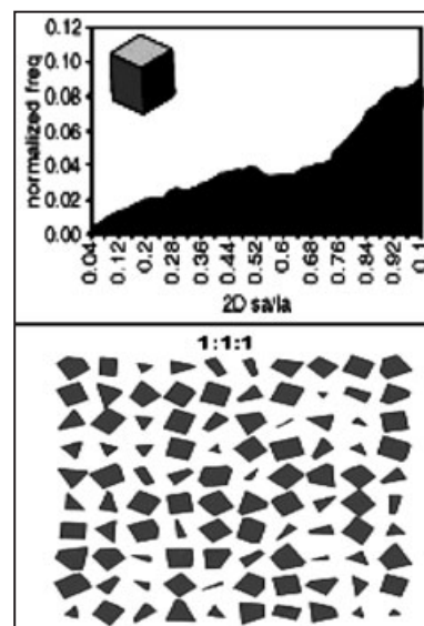
شکل ۴- نمودار نسبت عرض به طول برای بلور منشوری (Morgan & jerram, 2006)
