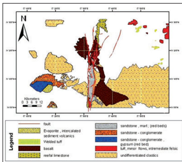
شکل ۲- نقشه زمین شناسی منطقه گندم بریان (برگرفته از نقشه ۱/۱۰۰۰۰۰ ناحیه لکر کوه، سایت سازمان زمین شناسی و اکتشافات معدنی کشور، www.GSI.ir)
