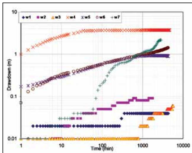
شکل ۵- نمودارهای افت- زمان آزمایش پمپاژ چاه‌های آهکی منطقه مورد مطالعه
