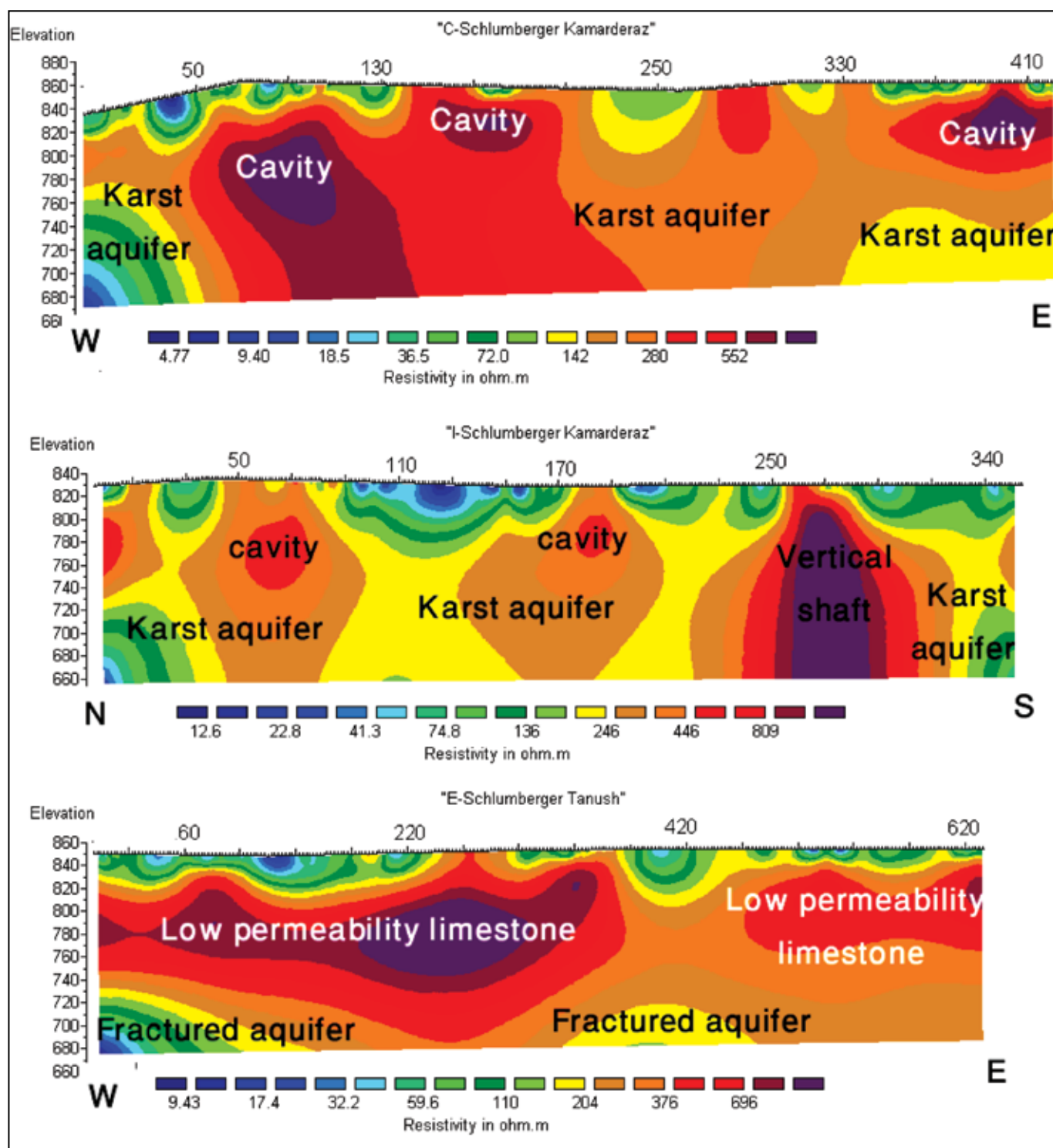
شکل ۹- مقاطع توموگرافی مقاومت الکتریکی حاصل از VES در نیمرخ های C و I (سازند آسماری) و E (سازند ایلام - سروک)
