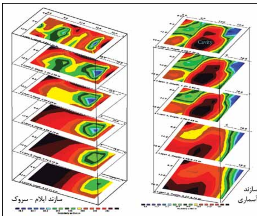
شکل ۱۳- توموگرافی مقاومت الکتریکی سه بعدی در آهک آسماری و آهک ایلام - سروک
