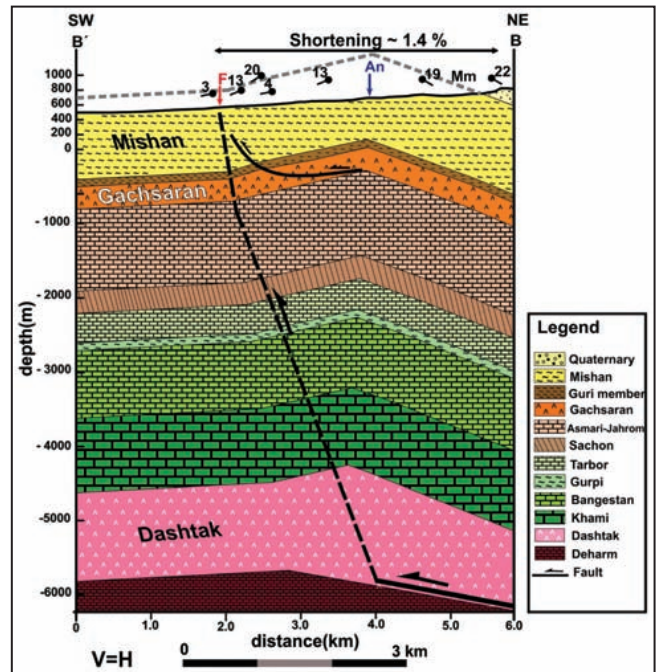
شکل ۴- برش ساختاری عمود بر تاق‌دیس هرمود. مسیر برش به صورت B-B' در شکل ۱ نشان داده شده است. بر روی این برش دو فرض ممکن در مورد منشأ گسل هرمود (ریشه گرفتن از گچساران یا دشتک؟) نمایش داده شده است. ستریای سازندها از نقشه ۱/۱۰۰۰۰۰ لار برداشت شده است.
