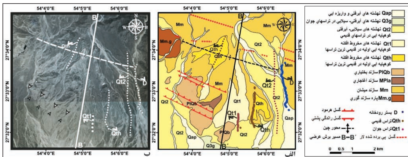
شکل ۳- الف) نقشه نوزمین‌ساخت تهیه شده بر روی تاقدیس هرمود (محدوده نقشه بر روی شکل ۱ نشان داده شده است). مسیرهای پیمایش شده با GPS کینماتیک بر روی پادگانه‌ها و رودخانه با نقاط به هم پیوسته نشان داده شده‌اند. مسیرهای نشان داده شده با نقطه‌چین از روی تصویر DEM برداشت شده‌اند. نیم‌رخ طولی نقاط پیمایش شده در شکل ۶ نشان داده شده است. ب) عکس هوایی مربوط به همان محدوده. مثلث‌های سفید رنگ بر روی عکس هوایی، مسیر گسل را نشان می‌دهند.
