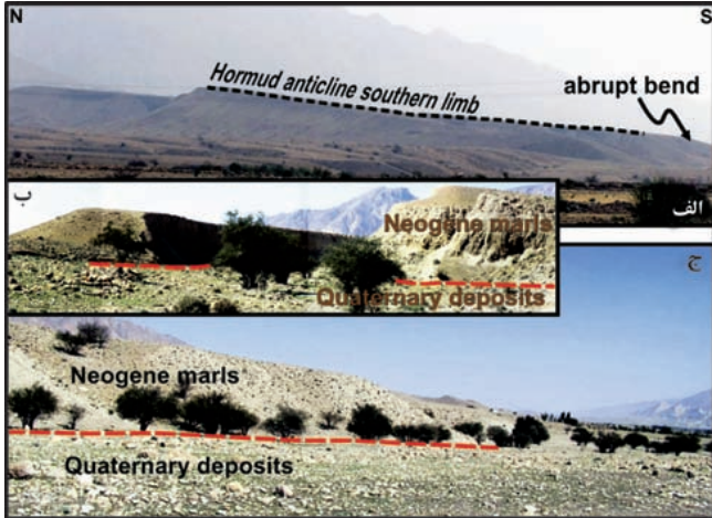
شکل ۵- الف) خمش ناگهانی و کوژی محلی در انتهای یال جنوبی تاق‌دیس هرمود که نشان‌دهنده محل گسل هرمود است. ب و ج) رد گسیختگی گسل هرمود در یال جنوبی تاق‌دیس هرمود در محل همبری ناگهانی میان مارن‌های نوژن در فرادپواره با نهشته‌های جوان کواترنر در فرودپواره (دید به سمت خاور).
