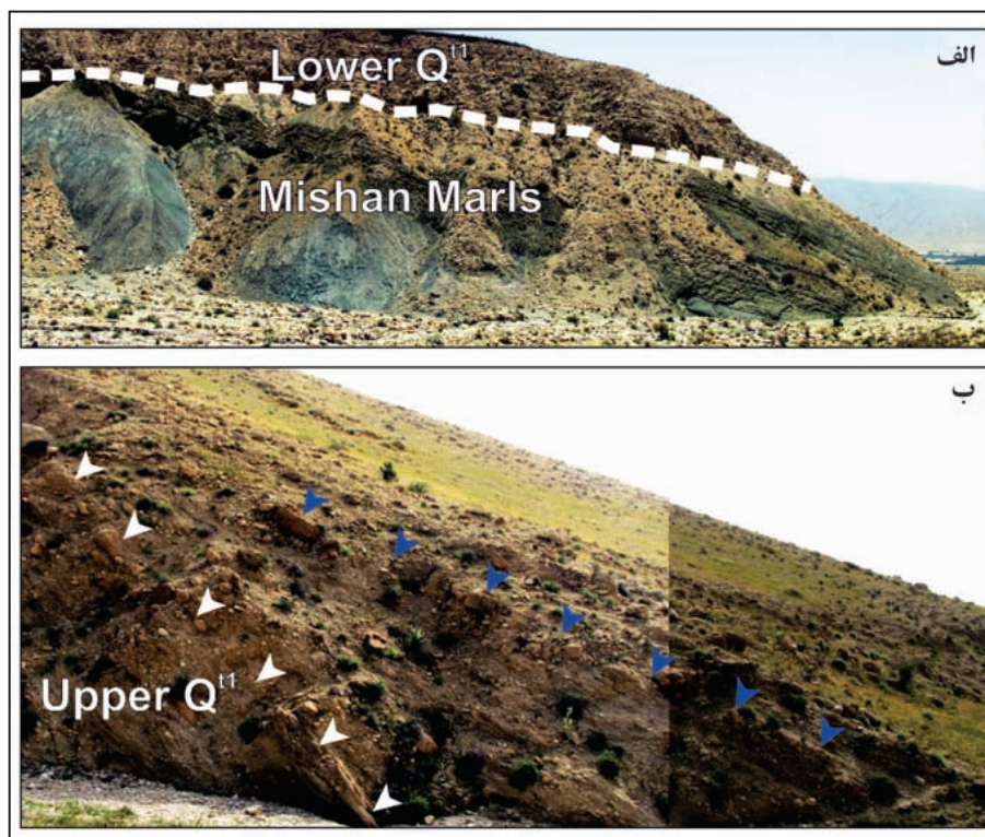
شکل ۸- الف) دگرشیبی بین مارن‌های میشان و بخش پایینی Q^1 . ستبرای بخش پایینی Q^1 در کل عرض تاقدیس یکسان است. ب) تفاوت تدریجی در میزان کج‌شدگی لایه‌بندی ضعیف در بخش بالایی واحد Q^1 که نشان‌دهنده همزمان با زمین‌ساخت بودن این واحد است (دید در هر دو تصویر به سمت خاور).
