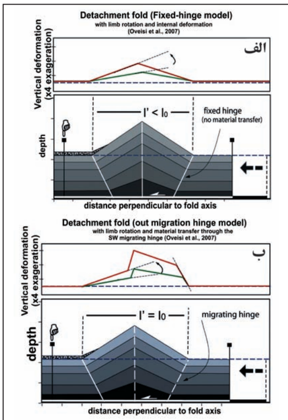
شکل ۷- مدل‌های مختلف چین‌های فراکنشی که با چرخش دامنه‌ای همراه شده‌اند. الف) چرخش دامنه‌ای با لولای ثابت همراه با تغییرشکل داخلی. ب) چرخش دامنه‌ای با مهاجرت لولای بیرونی و تغییرشکل ناودیسسی (Oveisi et al., 2007).
