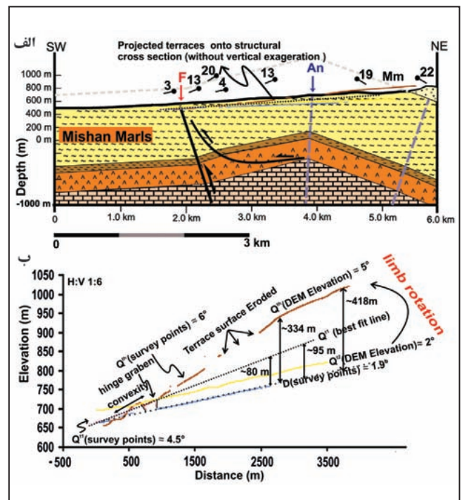
شکل ۶- الف) بخش بالایی برش ساختاری تاق‌دیس هرمود. نقاط پیمایش شده با GPS کینماتیک بدون بزرگنمایی عمودی بر روی برش پیاده شده‌اند. ب) نقاط پیمایش شده در عرض تاق‌دیس با بزرگنمایی عمودی ۶ برابر.
