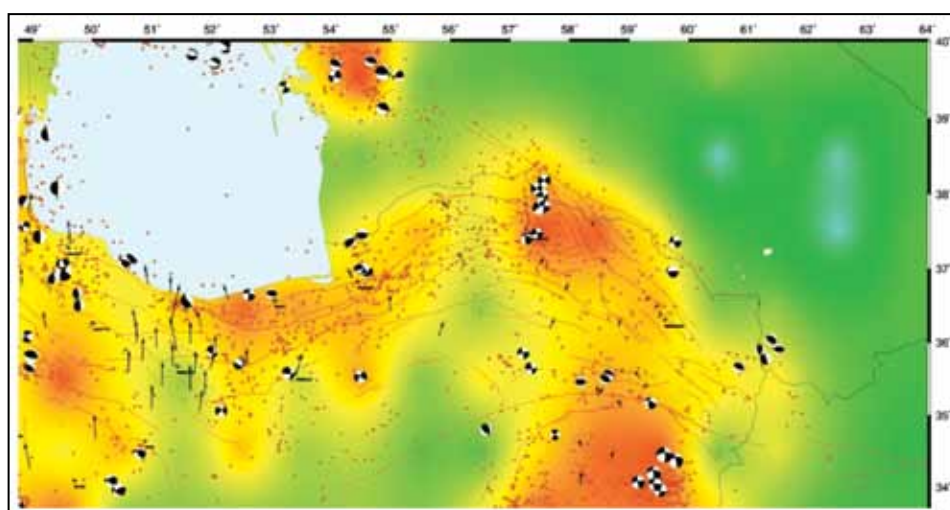
شکل ۸- گشتاور لرزه‌ای آزاد شده ناشی از رویداد زمین‌لرزه‌های دستگاهی و تاریخی. ساز و کار زمین‌لرزه‌ها مشابه شکل ۱ است. بردارها مقادیر نسبی سرعت ایستگاه‌های جی پی اس را نشان می‌دهد.
