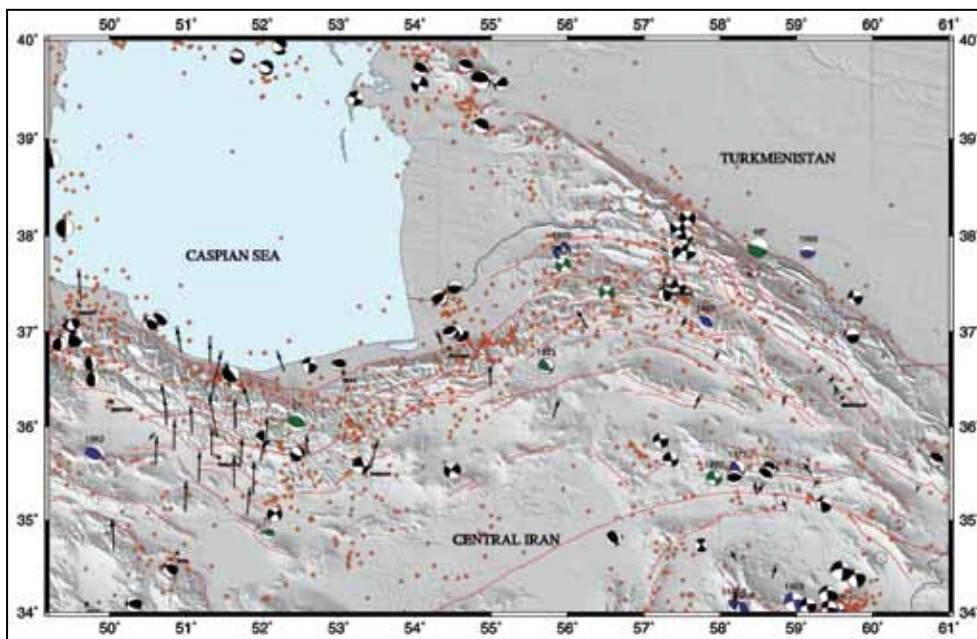
شکل ۱- گسل‌های اصلی لرزه‌زا و وضعیت لرزه‌خیزی منطقه. سازوکار کانونی زمین‌لرزه‌ها برگرفته از دانشگاه هاروارد (به رنگ سیاه)، مدل‌سازی امواج (آبی) و یا بر اساس قطبیت امواج اولیه (سبز) است. بردارها سرعت حرکت ایستگاه‌های جی‌پی‌اس را نشان می‌دهد. رومرکز سایر زمین‌لرزه‌ها با نقاط نارنجی رنگ نشان داده شده است.
