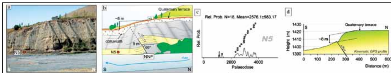
شکل ۳- مطالعات هندسه گسل و سن‌یابی بر روی گسل شمال نیشابور (Hollingsworth, 2006)
