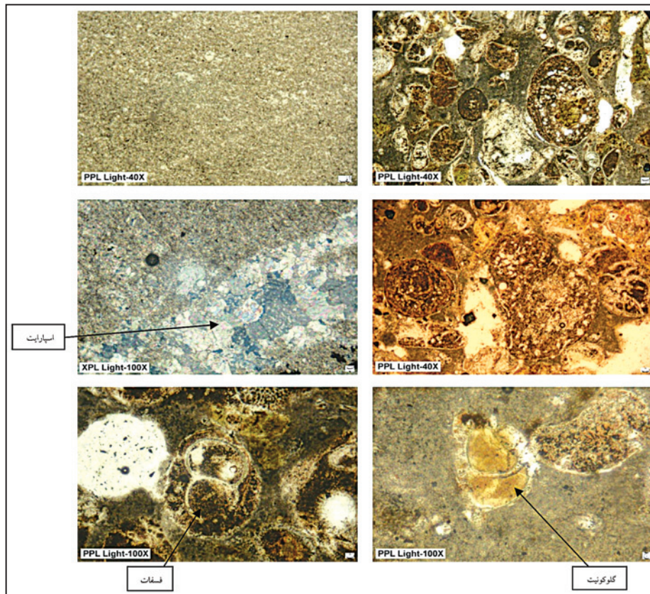
شکل ۵- ویژگی‌های دیده‌شده در مقاطع نازک. الف) میکرایت؛ ب) فسفاتیک بایومیکرایت؛ پ) تبدیل میکرایت به اسپارایت؛ ت) آلایت و پلت فسفات؛ ث) فسفات به شکل پرکننده حجرات که خود هسته آلایت شده است؛ ج) گلوکونیت در حجره فسیلی.
