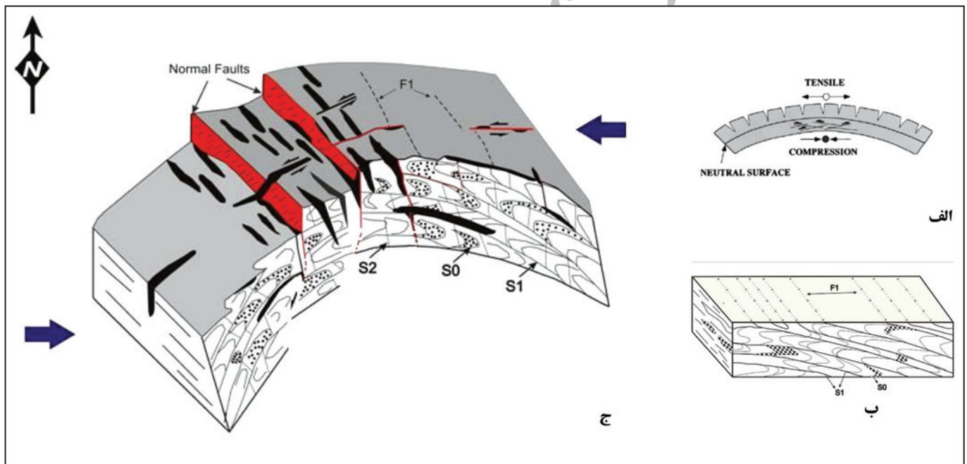
شکل ۸- الف) الگوی نمایشی از به‌وجود آمدن کشش عمود بر محور چین در بخش بیرونی طاق‌دیس و فشارش در بخش درونی طاق‌دیس را در سازوکار چین‌خوردگی کرنش طولی مماسی (Tangential Longitudinal Strain) نشان می‌دهد؛ ب) چین‌خوردگی خوابیده لایه‌بندی اولیه در مرحله نخست و به‌وجود آمدن برگوارگی مرحله اول؛ ج) چین‌خوردگی لایه‌بندی اولیه و برگوارگی مرحله اول به صورت چین‌های بسته تا باز ایستاده با سازوکار چین‌خوردگی کرنش طولی مماسی و به‌وجود آمدن درزه‌های کششی، گسل‌های عادی در بخش بیرونی طاق‌دیس و پر شدن آنها با کوارتز حاوی طلا.
