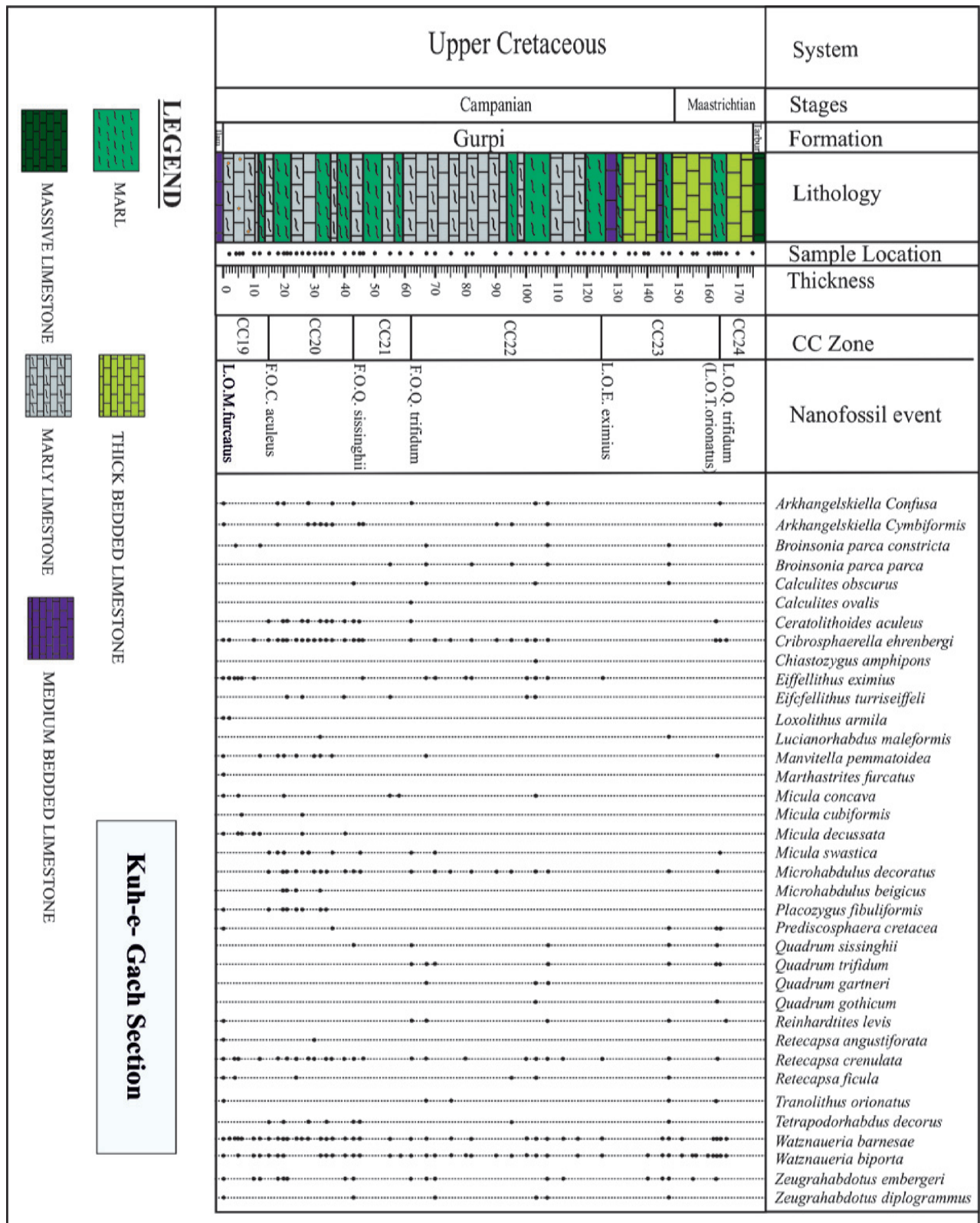
شکل ۳- زیست‌چینه‌شناسی سازند گورپی در برش کوه گچ بر مبنای نانوپروکون‌های آمکی.
