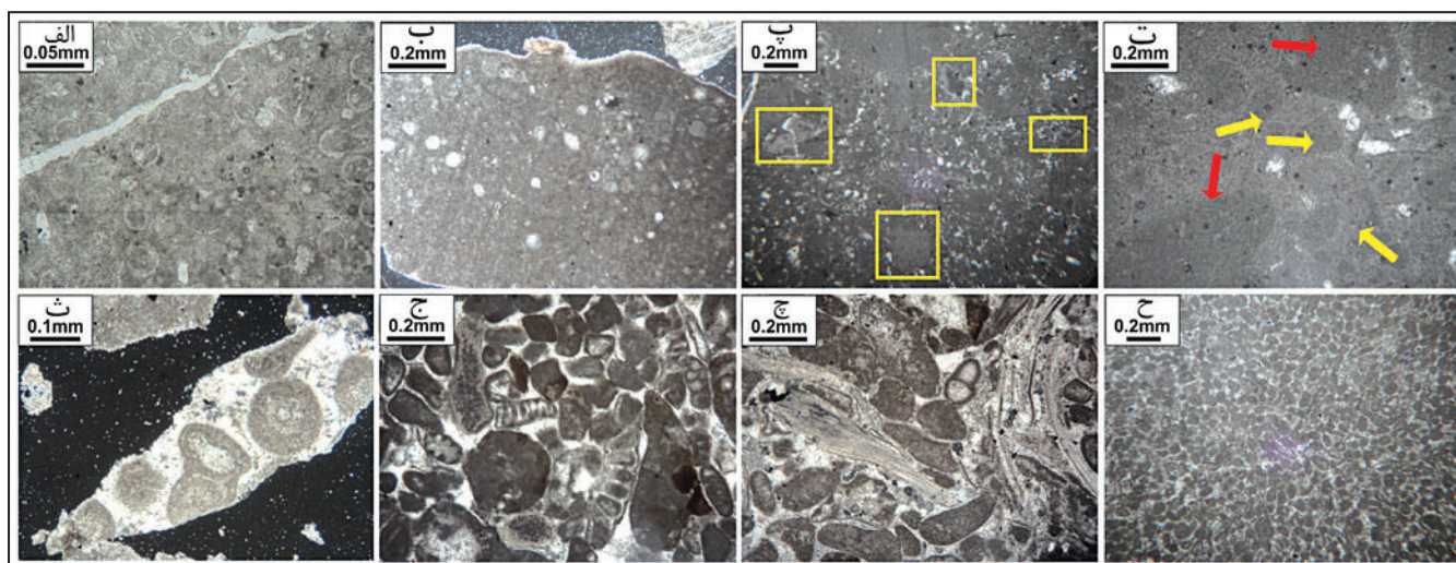
شکل ۳- مجموعه رخساره‌های محیط دریای باز و پشته‌های سدی (XPL به جز شکل الف). الف) پکستون کالیپونل دار (PPL)، چاه قزل‌تپه ۲، عمق ۱۸۶۲۰؛ ب) مادستون /وکستون کلسی اسفردار، چاه قزل‌تپه ۲، عمق ۱۸۵۰۰؛ پ) وکستون /مادستون بیوکلسی، کادرها قطعات اکتینوئید را نشان می‌دهند، برش چشمه‌خان؛ ت) وکستون اینتراکلسی حاوی پلویید، اینتراکلست گلی (فلش قرمز) و پلویید (فلش زرد) به سختی از زمینه میکریتی قابل تشخیص هستند، برش چشمه‌خان؛ ث) گرینستون آئیدی، چاه قزل‌تپه ۲، عمق ۱۸۴۴۰؛ ج) گرینستون اینتراکلسی حاوی پلویید، برش چشمه‌خان؛ چ) گرینستون پلوییدی اینتراکلسی حاوی بیوکلست، برش چشمه‌خان؛ ح) رخساره گرینستون /پکستون پلوییدی، برش چشمه‌خان.
