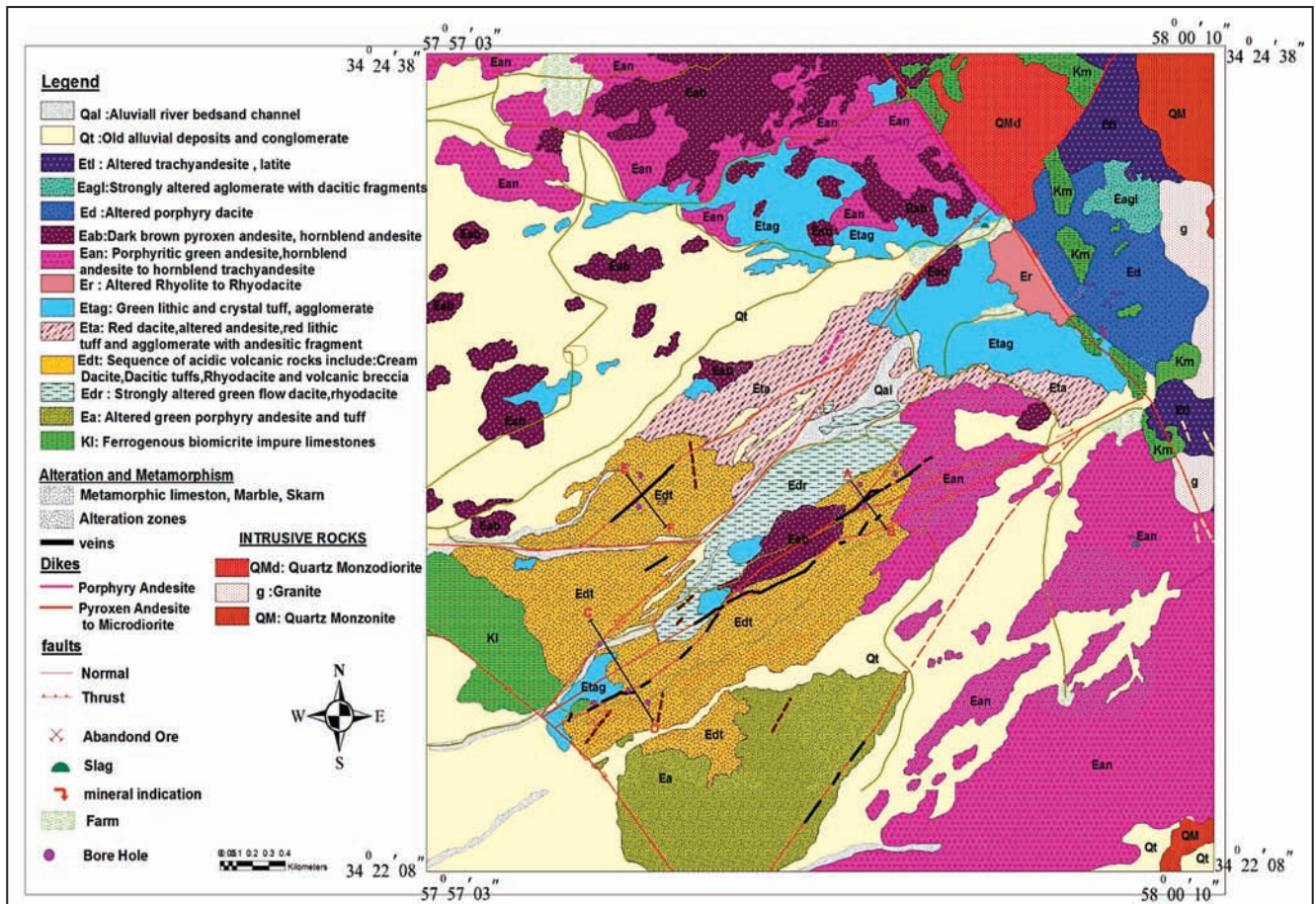
شکل ۲- نقشه زمین‌شناسی محدوده مورد مطالعه که در آن رگه‌های کانی‌سازی، نقاط حفاری و مقاطع عرضی مشخص شده‌اند.
