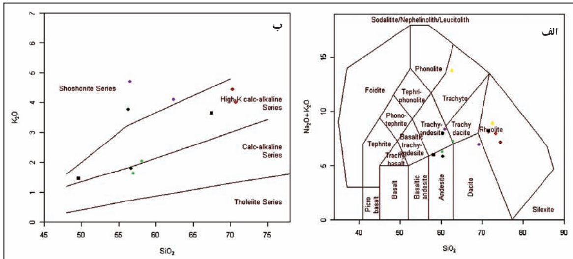
شکل ۳- الف) رده بندی سنگ های آتشفشانی میزان کانه زایی بر پایه SiO_2-Na_2O+K_2O (Middlemost, 1985); ب) نمودار تعیین سری ماگمایی سنگ های آتشفشانی میزان کانه زایی بر پایه SiO_2-K_2O (Peccerillo & Taylor, 1976).
