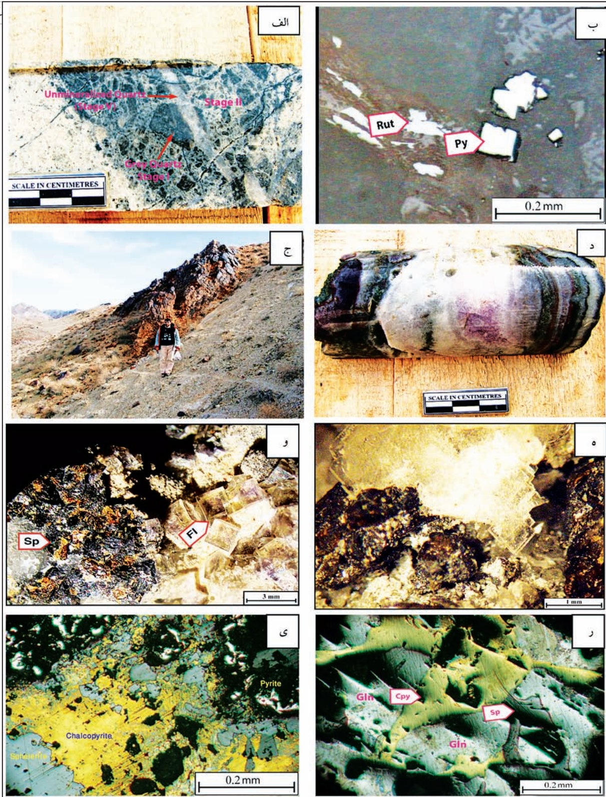
شکل ۷- الف) برش‌های گرمایی که در آن سیلیس‌های خاکستری تیره نسل اول، برشی شده و فضای بین پرش‌ها توسط سیلیس‌های نسل دوم پر و در مراحل بعدی توسط رگچه‌های سیلیسی نابارور نسل پنجم قطع شده‌اند؛ ب) پیریت‌های نیمه‌شکل‌دار تا کاملاً شکل‌دار ریزدانه نسل اول در کنار روتیل؛ ج) رخنمون‌هایی از رگه‌های سیلیسی-کربناتی دارای کان‌زایی در نسل دوم کان‌زایی (دید به سوی جنوب خاوری)؛ د) بافت‌های نواری-کلوفرم مربوط به مرحله دوم کان‌زایی در نمونه‌های به‌دست آمده از مغزه‌های حفاری؛ و) رگچه‌های دارای اسفالریت به رنگ قهوه‌ای با جلای صمغی همراه با فلوریت‌های کوبیک مربوط به مرحله دوم کان‌زایی؛ ه) حضور کلسیت‌های ورقه‌ای در کنار اسفالریت‌های تشکیل شده در مرحله دوم کان‌زایی؛ ی) کان‌زایی اسفالریت مربوط به مرحله دوم کان‌زایی که توسط کالکوپیریت و پیریت جایگزین شده است؛ ر) هم‌رشدی کان‌های اسفالریت، گالن و کالکوپیریت مربوط به مرحله دوم. کان فلوریت: Fl؛ اسفالریت: Sp؛ گالن: Gln؛ پیریت: Py؛ روتیل: Rut.
