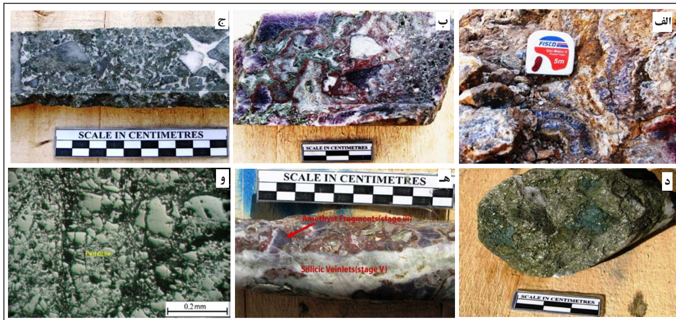
شکل ۸- الف) رگه‌های سیلیسی آمیستی مرحله سوم کانه‌زایی؛ ب) آمیست‌های مرحله سوم کانه‌زایی که در مراحل بعدی برشی شده‌اند؛ ج) برش‌های گرمایی مربوط به مرحله چهارم کانه‌زایی؛ د) کانه‌زایی سولفیدی دارای پیریت و پیروتیت در مرحله چهارم کانه‌زایی؛ ه) برش‌های دارای قطعات آمیستی مرحله سوم که در مرحله پنجم توسط سیلیس‌های شیری رنگ نابارور قطع شده است. و) کانه‌های پیروتیت مربوط به مرحله چهارم کانه‌زایی که در مراحل بعدی برشی شده است.
