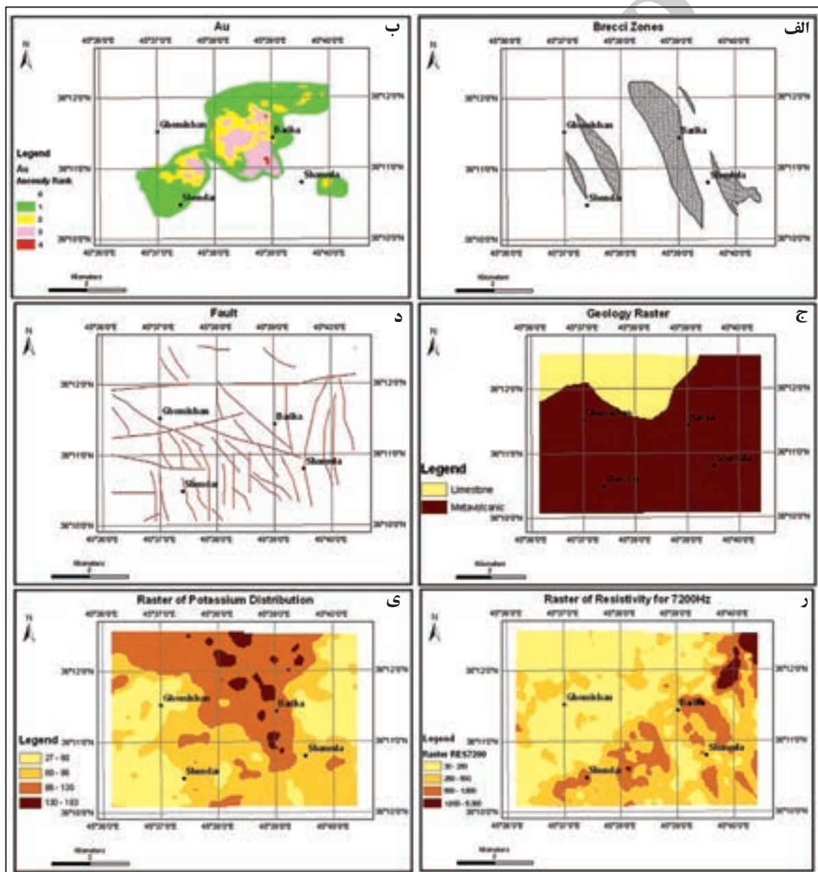
شکل ۲- نقشه پراکندگی پارامترهای مهم در کانی‌سازی طلای بی‌هنجاری باریکا؛ الف) بهنه‌های بُرشی؛ ب) پراکندگی عنصر طلا در برداشت‌های لیتوژئوشیمیایی؛ ج) واحدهای آهکی کرتاسه (رنگ روشن) و متاولکانیک کرتاسه (رنگ تیره)؛ د) پراکندگی خطواره‌های به‌دست آمده از داده‌های مغناطیس‌سنجی؛ ر) پراکندگی مقاومت ویژه الکتریکی به‌دست آمده از داده‌های الکترومغناطیس هواپرد؛ ی) پراکندگی رادیو عنصر پتاسیم.
