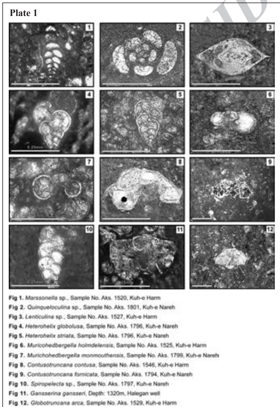
شکل ۵- معرفی زیست‌زون‌های برش کوه هرم، کوه نره و چاه‌ها لگان در مقایسه با زیست‌زون‌های Caron (1985) و Wynd (1965).
