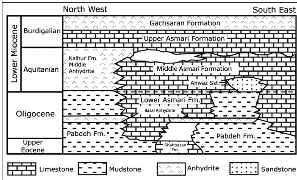
شکل ۴- بخش‌های سازند آسماری بر پایه سن و سنگواره‌ها در برش نمونه تنگ گل ترش در ناقدیس کوه آسماری (Mossadegh et al., 2009).
