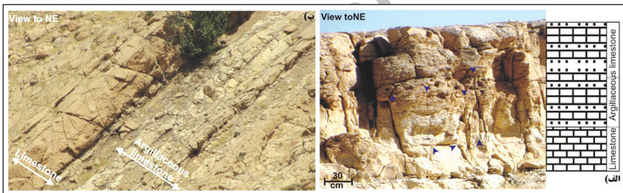
شکل ۵- واحدهای آهک و آهک رسی در پال پشانی ناقدیس کوه آسماری. الف) توقف گسترش عمودی شکستگی‌های در آهک‌های رسی مشخص است؛ ب) واحدهای آهک رسی به رنگ نخودی تا کرم روشن و آهک به رنگ قهوه‌ای تا قهوه‌ای تیره دیده می‌شوند.
