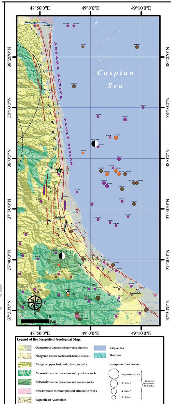
شکل ۲- نقشه لرزه‌زمین‌ساخت کوه‌های تالش. خطوط سرخ رنگ نشان‌دهنده شاخه‌های گسل و به ترتیب دوایر صورتی کم رنگ، سرخ رنگ، سبز، نارنجی و بنفش پررنگ نشان‌دهنده بزرگای زمین‌لرزه‌ای Ms، Ml و Mb هستند (Kaveh et al., 2013).
