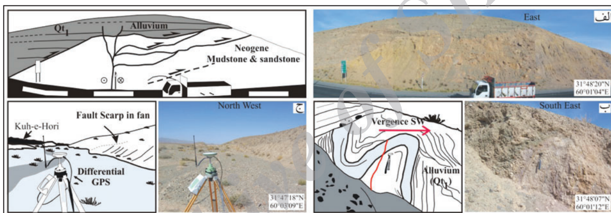
شکل ۵- الف) مقطعی از گسل شوسف در برش رسوبات مخروط افکنه‌ای در جاده شوسف- نهندان. گسل راندگی شوسف در واحدهای Qt 1 ، 35 NE، N290 اندازه‌گیری شده است. شکل‌گیری ساختار گلواره در رسوبات نوژن و قطع راندگی شوسف نشان از فعالیت امتدادلغز گسل به صورت محلی دارد؛ ب) چین خوردگی در واحدهای Qt 1 که سوی رانش جنوب باختری را نشان می‌دهد؛ ج) نمایی از پرتگاه گسلی شوسف در رسوبات مخروط افکنه Qt 1 (GPS تفاضلی به عنوان مقیاس). موقعیت شکل‌های بالا در تصویر ماهواره‌ای شکل ۴- ب آمده است.
