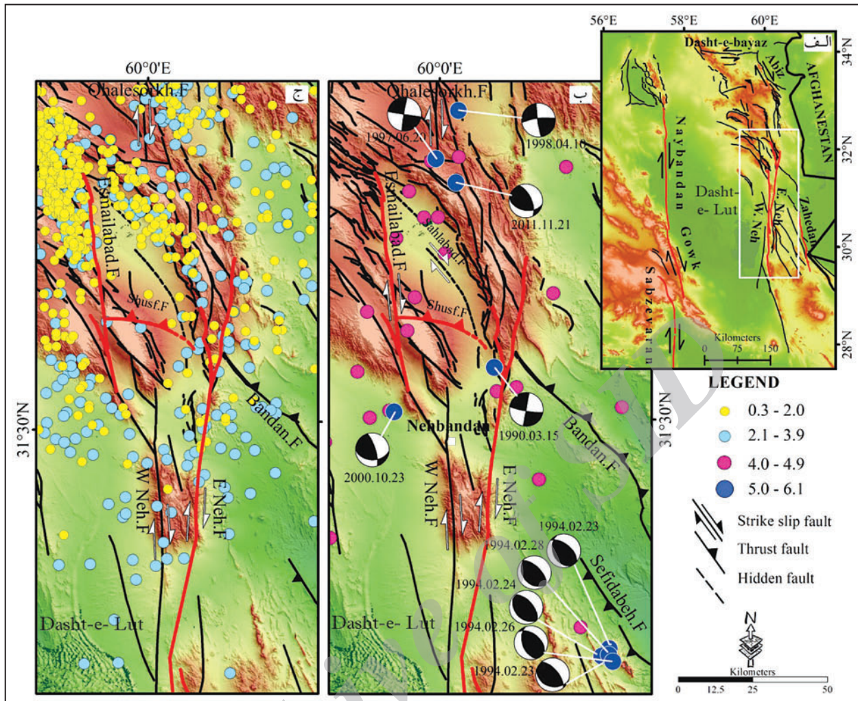
شکل ۲- الف) سامانه گسلی سیستم و نایند مرزهای خاوری و باختری بلوک لوت را تشکیل می‌دهند. کادر سفید رنگ موقعیت گستره شوسف در سامانه گسلی سیستم را نمایش می‌دهد؛ ب) زمین‌لرزه‌های دستگاهی ثبت شده با بزرگی بالای ۴. دوایر آبی کانون سطحی زمین لرزه‌های بزرگ‌تر از ۵ به همراه سازوکار کانونی آنها را نشان می‌دهد (ماخذ: جدول ۱)؛ ج) رویدادهای خردلرزه‌ای در فاصله زمانی ۲۰۱۴-۲۰۰۶ (IGUT) نشان از فعالیت سامانه‌های گسلی شمالی- جنوبی و پایانه‌های آنها در گستره مورد مطالعه دارد. خطوط سیاه گسل‌های فعال در منطقه و خطوط سرخ سامانه گسلی مورد نظر در این پژوهش بوده که سبب ایجاد فراگام گرفتاری نه خاوری- اسماعیل‌آباد شده است.
