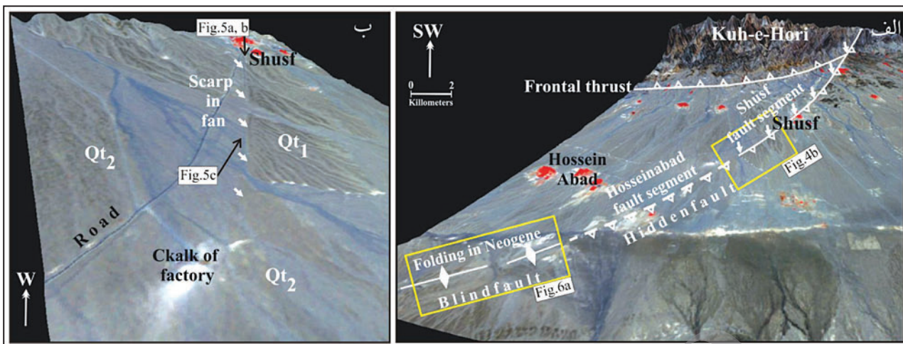
شکل ۴- الف) تصویر ماهواره‌ای Aster3D از گستره شوسف. در این تصویر اثر پرتگاه قطعه گسلی شوسف به صورت بریدگی در کوهستان و مخروط افکنه قدیمی (پیکان سفید) و نیز قطعات پنهان و کور راندگی شوسف در تصویر ماهواره‌ای به صورت بریدگی در مخروط افکنه قدیمی (Qt 1 ) نمایان است (پیکان سفید).
