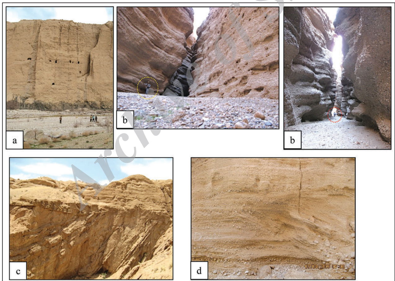
شکل ۴- تصاویری از وضعیت نهشته‌های آبرفتی کهن (Qt1) که در قالب بادزن‌های کهن در صحرا مشاهده می‌شود؛ (a) پادگانه آبرفتی در دیواره رودخانه سردر که به صورت دگرشیب بر روی نهشته‌های تیره رنگ دونین-کرنیفر برجای گذاشته شده است (حفرات مشاهده شده، غارهای باستانی برخاسته معروف به خانه گبر می‌باشند) - خاور طبس؛ (b) دو نمونه از تنگ‌دره‌های ایجاد شده توسط رودخانه سردر در نهشته‌های آبرفتی بادزن‌های کهن به صورت دره آبگذر پیشین - خاور طبس؛ (c) قرارگیری نهشته‌های آبرفتی کهن به صورت دگرشیب بر روی رسوبات نوژن - دیواره کال جنی، شمال باختری طبس؛ (d) وضعیت دانه‌بندی و طبقه‌بندی چلیپایی در رسوبات آبرفتی کهن - دیواره کال جنی، شمال باختری طبس.
