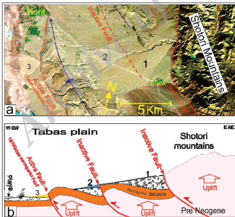
شکل ۶- (a) تصویر ماهواره‌ای از گسل‌های غیر پویا (یا با جنبش کم) و گسل جدید (گسل زمین‌لرزه سال ۱۳۵۷ طبس) و سه نسل بادزن آبرفتی ایجاد شده در بخش‌های میانی دشت طبس، به جایگاه چین‌خوردگی‌های نئوژن و گسل‌ها نسبت به بادزن‌های آبرفتی دقت شود؛ (b) برش نمادین (بدون مقیاس) از وضعیت شکل ۶-ا، در اثر پیشروی پیشانی جنبش‌های ساختاری، یک ساختمان فلسی ایجاد شده و در این حالت کوهستان شتری و مجموعه بادزن‌های نسل ۱ و ۲ به صورت یکپارچه در حال فراخاست هستند. برای موقعیت جغرافیایی، به شکل ۲ مراجعه شود.
