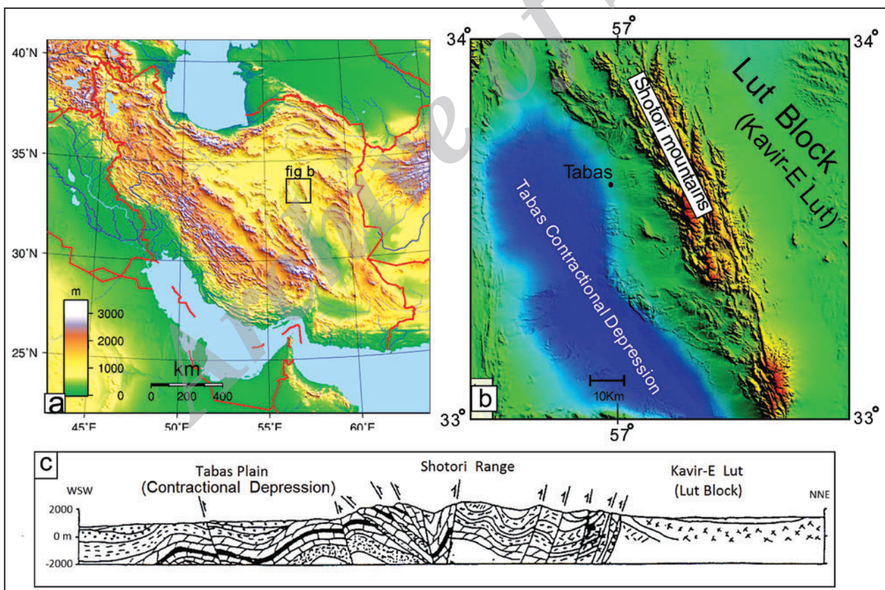
شکل ۱- a, b) تصویر DEM (با دقت ۸۰ متری) از موقعیت کوهستان شتری در خاور ایران به‌صورت یک سیمای زمین‌ریختی برجسته بر حداصل کویر لوت و فروافتادگی فشارشی دشت طبس؛ c) گسل ساخت مثبت (ساخت نخلی) در برش ساختاری از کوهستان شتری (اشتوکلین و نبوی، ۱۳۴۸- با اصلاحات).
