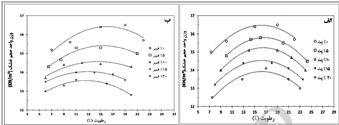
شکل ۵- منحنی‌های تراکم خاک ماسه‌ای با اختلاط الف) خرده‌های بطری؛ ب) فیبر لاستیک.
