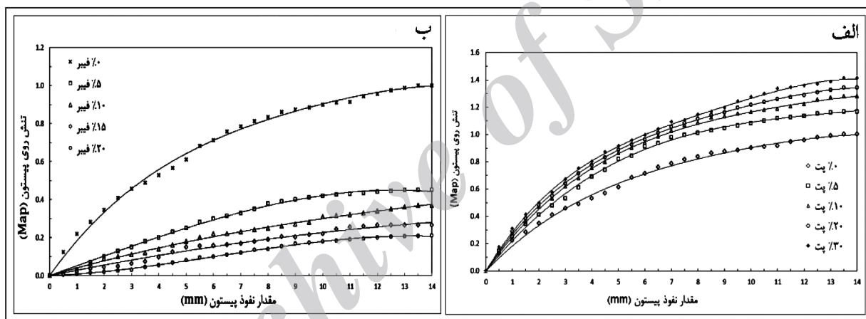
شکل ۶- منحنی نسبت باربری کالیفرنیای مخلوط ماسه با الف) خرده‌های بطری؛ ب) فیبر لاستیک فرسوده.
