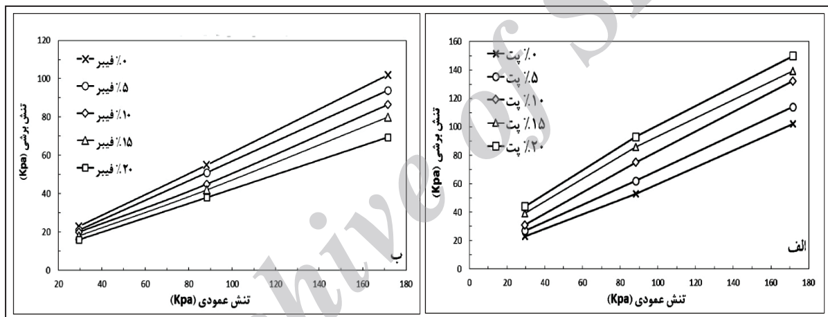
شکل ۱۰- تغییرات تنش برشی پیشینه در درصد اختلاط‌های مختلف الف) پت؛ ب) فیبر.
