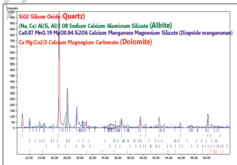
شکل ۴- پیک تجزیه XRD و کانی‌شناسی خاک ماسه‌ای.
