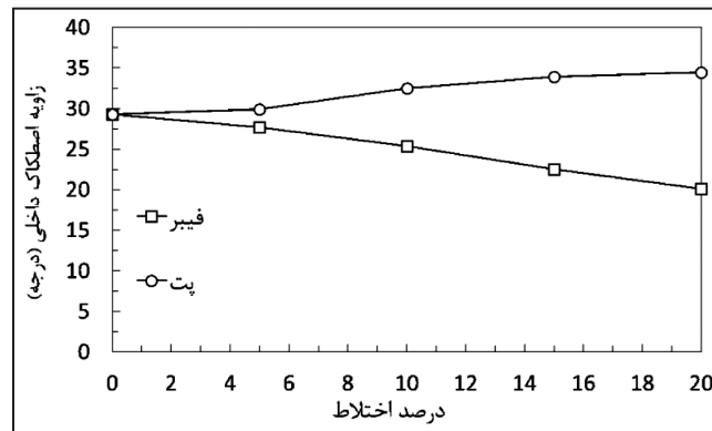
شکل ۹- تغییرات زاویه اصطکاک داخلی در نتیجه افزایش درصد اختلاط مواد افزودنی.
