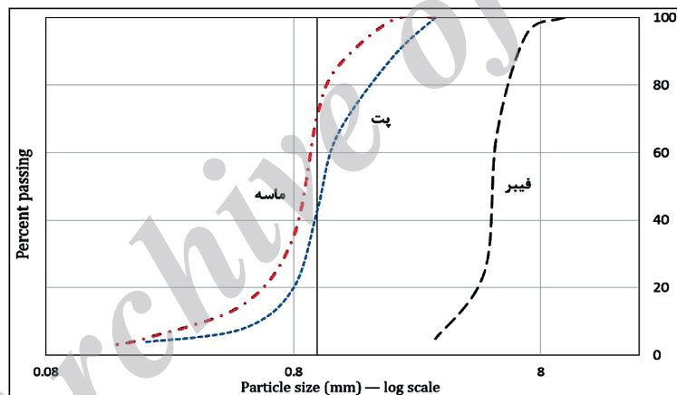
شکل ۳- نمودار دانه‌بندی مصالح ماسه‌ای، خرده‌های بطری و فیبر لاستیک فرسوده.
