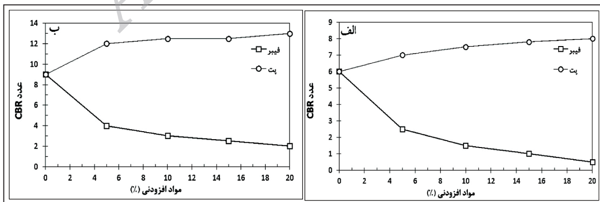
شکل ۱۱- تغییرات عدد CBR در درصد‌های اختلاط از مواد افزودنی در مقدار نفوذهای الف) ۲/۵ میلی‌متر؛ ب) ۵ میلی‌متر.
