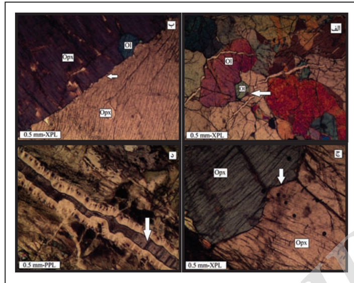
شکل ۵- شواهد میکروسکوپی سازوکار انتقال توده پراکنده در مجموعه ده‌شیخ. الف) تماس دانه‌ای فرورفته میان بلورهای الیون در لرزولیت؛ ب) تماس دانه‌ای لبه صاف شده میان بلورهای ارتوپروکسن در ارتوپروکسنیت؛ ج) تماس دانه‌ای نفوذی به درون میان بلورهای ارتوپروکسن در ارتوپروکسنیت؛ د) رگچه کربناته فیبری (پیکان سفید رنگ) در هارزبورژیت، سرپانتین‌های بلوکی در حاشیه رگچه دیده می‌شوند.
