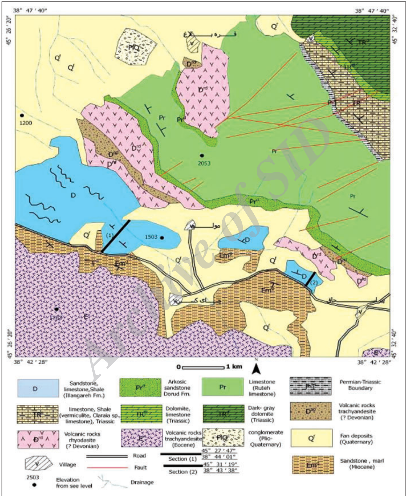
شکل ۴- نقشه زمین‌شناسی برش مرکب پیراسحاق، رسم دوباره از روی نقشه‌های زمین‌شناسی ۱:۱۰۰۰۰۰ جلغا (عبدالهی و حسینی، ۱۳۷۵) و قره ضیاء‌الدین (اسکویی و حاج علیلو، ۱۳۷۴).
