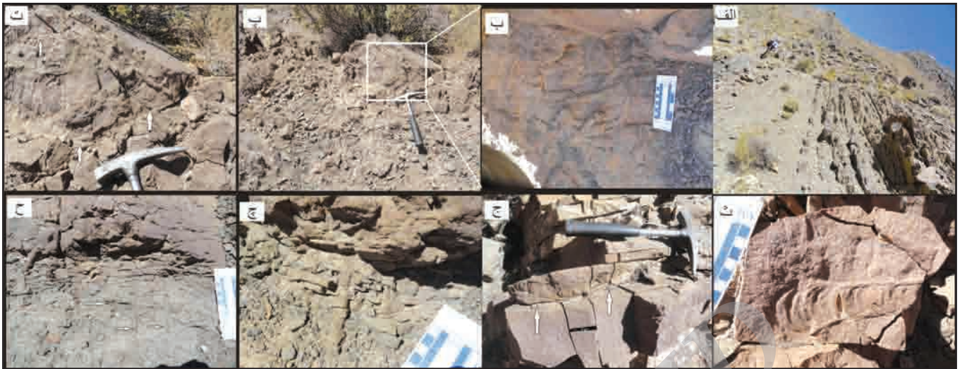
شکل ۹- الف) تصویر کلی از رخساره (dLSF) dista lower shoreface؛ ب) Rhizocorallium irregula ؛ پ، ت و ث) Rhizocorallium jenese ؛ ج) Rhizocorallium irregula موازی با سطح چین‌بندی؛ چ و ح) Ophiomorpha .
