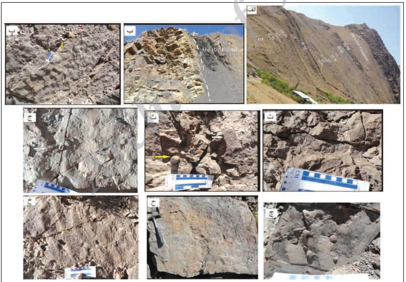
شکل ۱۰- الف) تصویر کلی از مجموع توالی رخساره‌های بخش دریایی باز تحت تأثیر امواج سازند نایبند - offshore (ot), offshore transition (ot), dista lower shoreface (dLSF), proximal lower shoreface (pSFL), proximal lower shoreface (pSFL)؛ ب) رخساره (shelf (of-sh)؛ ج) Palaeophycus و فسیل‌های پیکره‌ای؛ ت) Rhizocorallium jenese ؛ ث) Rhizocorallium ؛ ج) Monocraterion ؛ چ) Arenicolites ؛ ح) Ophiomorpha (پیکان زرد)؛ د) Arenicolites ؛ ه) Skolithos ؛ و) Palaeophycus ؛ ز) Monocraterion (پیکان زرد)؛ ح) Arenicolites و Skolithos با ساختارهای قائم از pipe-rock ichnofabric؛ ح) Arenicolites و Skolithos با ساختارهای قائم از pipe-rock ichnofabric؛ ح) Arenicolites و Skolithos (پیکان زرد)؛ ح) Palaeophycus و
