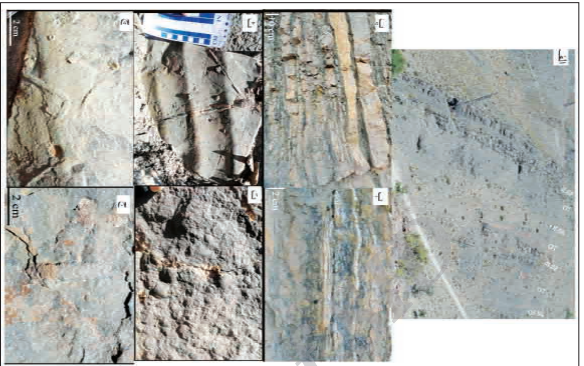
شکل ۸- الف) تصویر کلی از رخساره‌های بخش دریایی باز تحت تأثیر امواج distal lower shoreface (off-shore-shelf (of-sh) transition (ot), offshore-shelf (of-sh) transition (ot), offshore-shelf (of-sh) transition (ot))؛ ب) چینه‌بندی مورب هوموگی کوچک؛ مقیاس در لایه‌های باستانی؛ ب) چینه‌بندی مورب هوموگی بزرگ؛ مقیاس در لایه‌های باستانی؛ بیشتر از ۵ سانتی‌متر؛ ت) فسیل‌های پیکره‌های؛ ث) ریل موجی؛ با اثر فسیل Palaeophycus gyrochorte ؛ ج) Protovirgulatia
