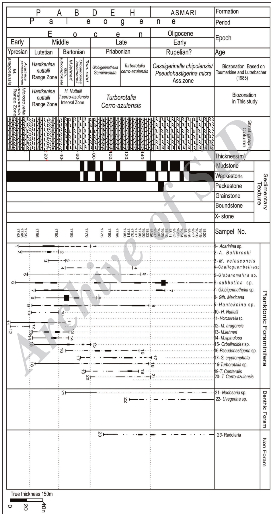
شکل ۳- ستون زینست چینهنگاری توالی سازند پاینده (الوسن میانی) - بالایی) در برش افشگر.
