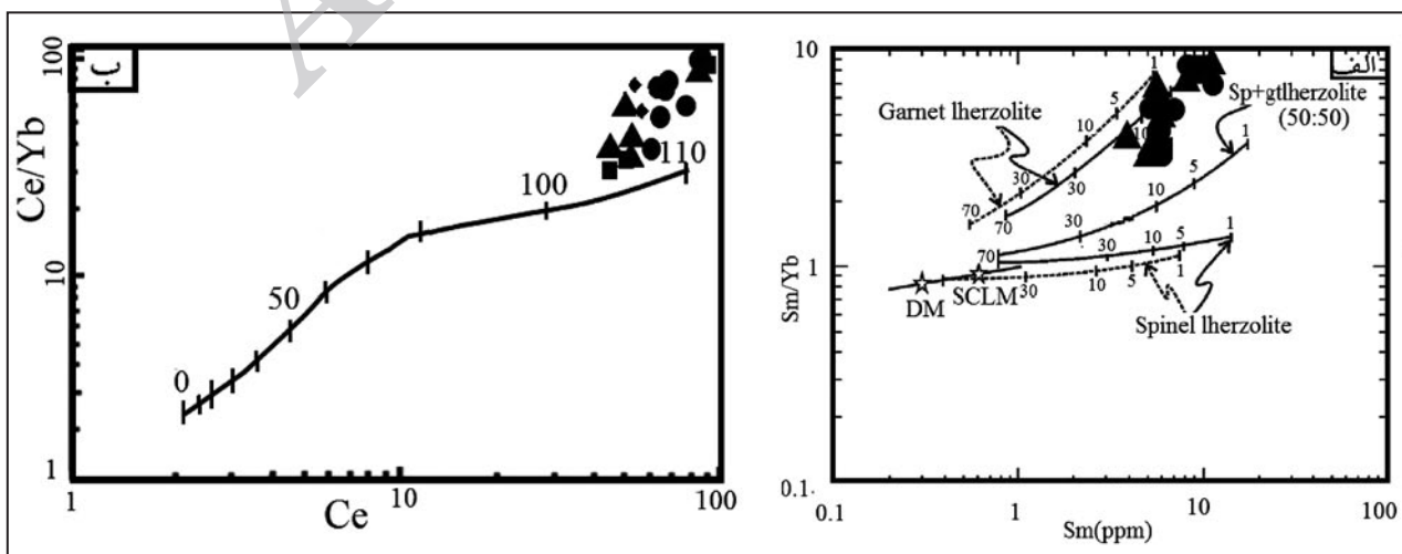
شکل ۱۷- موقعیت نمونه‌های بازالتی الیگوسن لبه شمالی ایران مرکزی در نمودارهای: الف) Sm/Yb در برابر Sm؛ ب) Ce/Yb در برابر Ce (Li & Chen, 2014).
