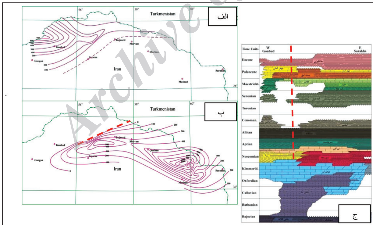
شکل ۱۲- نقشه تغییرات ستبرای سازندهای الف) زرد؛ ب) شوریجه (افشارحرب، ۱۳۷۳). خط چین سرخ رنگ محدوده گسل جوزک- قتلیش را نمایش می‌دهد؛ ج) تغییرات چینه‌شناسی کپهداغ از خاور به باختر (افشارحرب، ۱۳۷۳).
