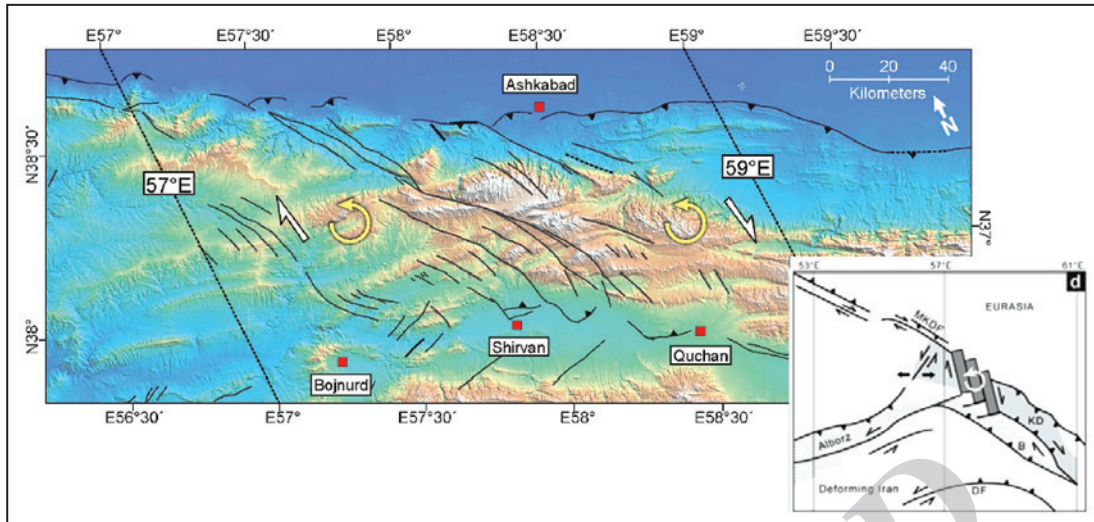
شکل ۳- نقشه توپوگرافی خاور محدوده مورد بررسی (میان طول‌های جغرافیایی ۵۷°E تا ۵۹°E). کوتاه‌شدگی در این بخش از کپه‌داغ به احتمال از راه چرخش پادساعت‌گرد بلوک‌هایی صورت می‌گیرد که با گسل‌های راست‌الغز راست‌بر در بر گرفته شده‌اند (Hollingsworth, 2007).
