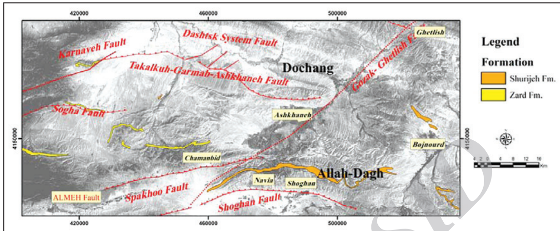
شکل ۱۱- گسترده سازی شوریجه و زرد در محدوده مورد بررسی نسبت به گسل جوزک- قتلیش روی تصویر ماهواره‌ای.
