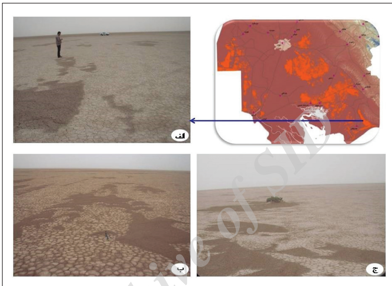
شکل ۱۲- کفه‌های رسی شرق هندوچان: الف، ب و ج) انتقال بخش‌های دانه‌ریز رسی و تشکیل برخان‌ها در نتیجه تجمع ذرات دانه‌درشت‌تر.
