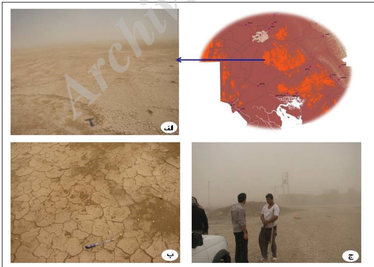
شکل ۹- پهنه رسی در باختر نهر مالچ در جنوب اهواز: الف) برداشت بخش‌هایی از خاک سطحی به ژرفای بیش از ۳ سانتی‌متر؛ ب) فسیل‌های شکم پا در نهشته‌های رسی؛ ج) رخداد توفان گردوغبار و غلظت بالای آن در آبادی‌های محدوده کانون.
