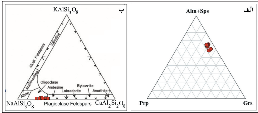
شکل ۶- الف) نمودار سه‌تایی مجموع اعضای پایانی Pry-(Alm-Sps)-Grs و موقعیت ترکیبی گارنت‌ها در گارنت آمفیبولیت‌های تجزیه شده روی آن؛ ب) موقعیت ترکیبی پلاژیو کلازهای تجزیه شده متعلق به نمونه‌های آمفیبولیتی مجموعه شترکوه روی نمودار سه‌تایی رده‌بندی فلدسپارها (Deer et al., 1992).
