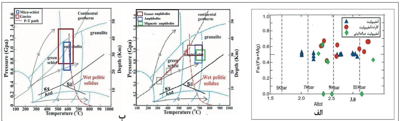
شکل ۸- الف) نمودار Al_{total} در برابر X_{Fe} آمفیبول (Schmidt, 1992)؛ ب) نمودار P-T برای گارنت آمفیبولیت‌های مورد مطالعه، نمونه‌های میکاشیستی و گارنت گنیسی و متابازیتی (کادرهای رنگی) در میدان پایداری کیانیت و مسیر دگرگونی پیش‌رونده که بر پایه محدوده‌های دما و فشار تعیین شده رسم شده است. دما و فشارهای به دست آمده شرایط رخساره آمفیبولیت تا آمفیبولیت بالای را برای متابازیت‌ها و متابلیت‌های مجموعه شترکوه نشان می‌دهد.
