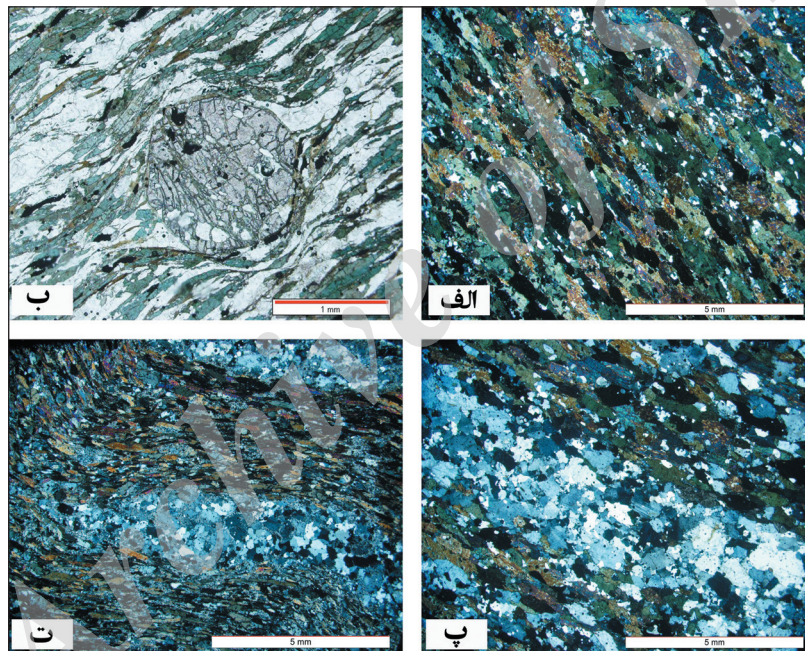
شکل ۴- الف) بافت نماتوبلاستی ناشی از حضور آمفیبول های سوزنی شکل به همراه پلاژیوکلازهای جهت یافته در هورنبلند شیست ها (XPL)؛ ب) پورفایروبلاست شکل دار گارنت دارای ادخال هایی از کوآرتز و بیوتیت. بافت پورفایروبلاستی این گارنت، ناشی از رشد پس از زمین ساخت آن است (PPL)؛ پ) تصویری از لایه های تیره و روشن در یک آمفیبول شیست میگماتیته شده (XPL)؛ ت) چین خوردگی در یک آمفیبول شیست میگماتیته شده (در مقیاس میکروسکوپی یا بسیار کوچک) (XPL).
