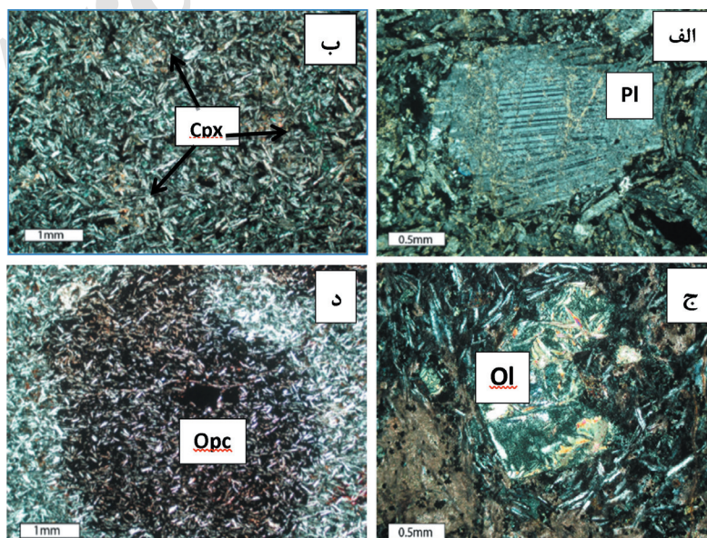
شکل ۳- (الف) بافت میکروولیتی پورفیری در سنگ‌های آتشفشانی مورد مطالعه؛ (ب) بافت اینترسترال که فضای میان میکروولیت‌های پلاژیوکلاز توسط بلورهای ریز کلینوپیکس پر شده است؛ (ج) قالب برجای مانده از الومین (Ol) که به‌طور کامل دگرسان شده است؛ (د) تمرکز بالای کانی‌های کدر (Opc) در بخش‌هایی از زمینه سنگ. همه تصاویر در حالت XPL.
