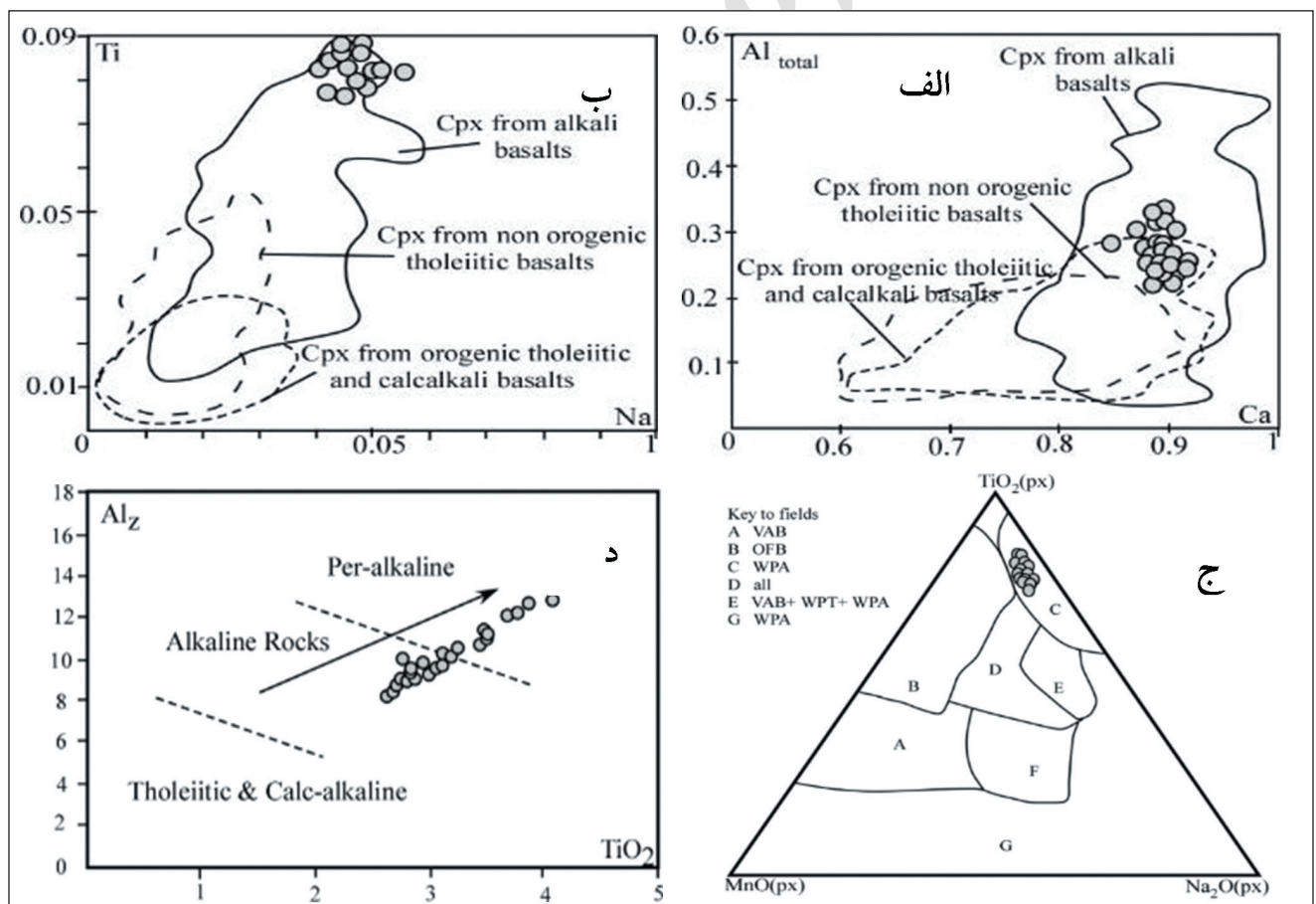
شکل ۷- نمودارهای تمایز سری‌های ماگمایی بر پایه ترکیب شیمیایی کلینوپروکسن؛ الف) نمودار تغییرات Al_{tot} در برابر Ca (Leterrier et al., 1982)؛ ب) نمودار تغییرات Ti در برابر Na (Leterrier et al., 1982)؛ ج) نمودار مثلثی TiO_2 -MnO-Na 2 O بر پایه ترکیب کلینوپروکسن (Nisbet and Pearce, 1977)؛ د) نمودار Al_z در برابر TiO_2 (Le Bas, 1962)؛ اختصارات بدین شرح است: بازالت‌های کمان آتشفشانی (VAB)، بازالت‌های کف اقیانوس (OFB)، بازالت‌های توله‌ایتی درون ورقه‌ای (WPT) و بازالت‌های آلکالن درون ورقه‌ای (WPA).
