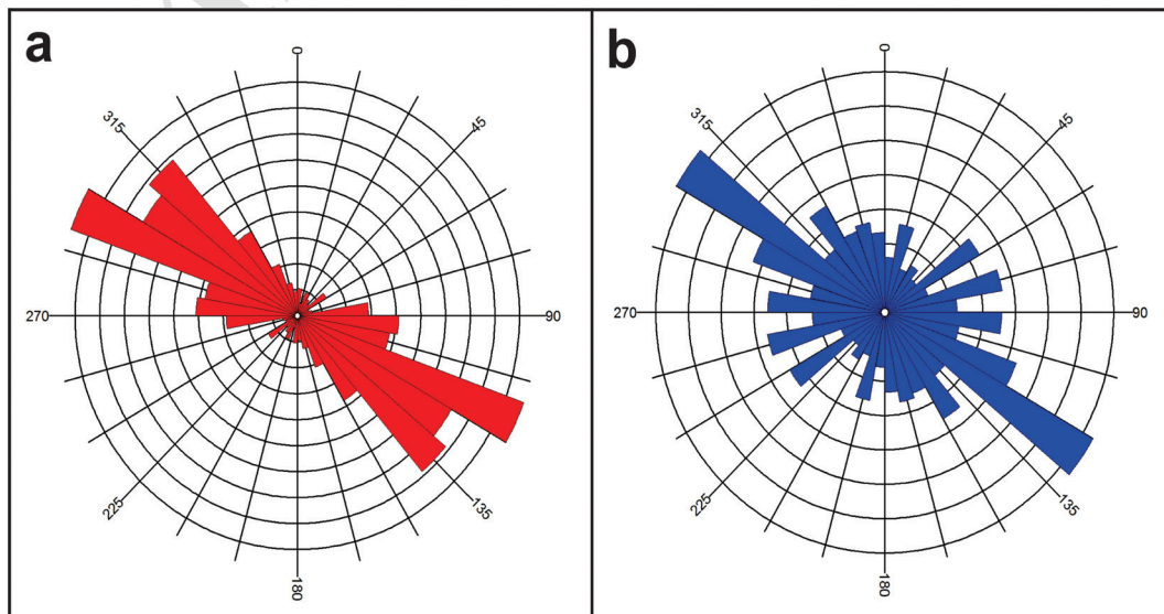
شکل ۷- نمودارهای گل سرخی نقشه کلی خطواره‌ها و گسل‌های منطقه آوج - آبرگرم؛ الف) نمودار گل سرخی مربوط به شبکه گسلی منطقه مورد مطالعه؛ ب) نمودار گل سرخی مربوط به خطواره‌های منطقه مورد مطالعه.
