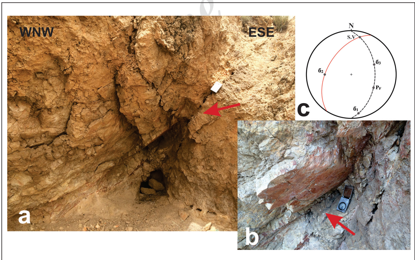
شکل ۱۱- الف) عملکرد گسل با موقعیت N30 / 50NW در سازند سلطانیه ناحیه کیسه‌چین؛ ب) این گسل خش‌لغزهایی با ریزک ۲۰ درجه شمالی دارد. پ) استریوپلات رسم شده که موقعیت محورهای اصلی تنش و سازوکار مورب‌لغز این گسل را نشان می‌دهد.
