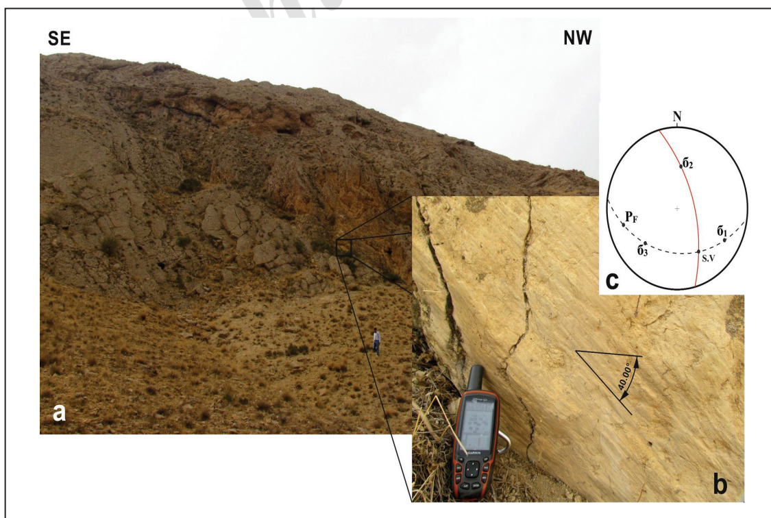
شکل ۹- صفحه گسلی، بخش یا قطعه جنوب باختری گسل حسن آباد؛ الف) عملکرد گسل با موقعیت N165 / 70NE ؛ ب) آینه گسل یاد شده که دارای خشن‌لغزهایی با ریک 40^{\circ} درجه از جنوب خاوری است؛ پ) استریوپلات رسم شده که موقعیت محوره‌های اصلی تنش و سازوکار مورب‌لغز این گسل را نشان می‌دهد.
