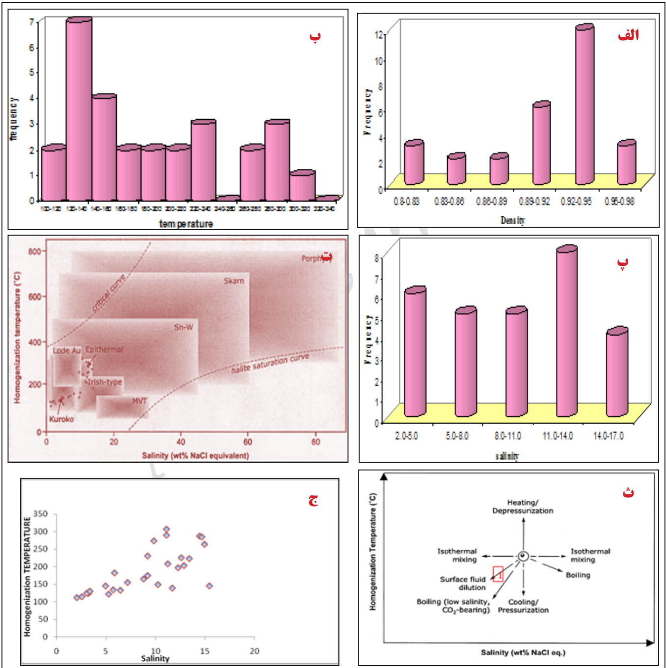
شکل ۱۱- الف) نمودار مقدار چگالی میانبره‌های سیال در برابر فراوانی آنها؛ ب) نمودار مقدار دمای همگن شدگی میانبره‌های سیال در برابر فراوانی آنها؛ پ) نمودار مقدار شوری میانبره‌های سیال در برابر فراوانی آنها؛ ت) دیاگرام شوری- دمای همگن شدن سیالات درگیر در انواع کانسارها (Wilkinson, 2001)، نقاطی که با دایره پررنگ نمایش داده شده مربوط به داده‌های به دست آمده از سیالات درگیر در محدوده مطالعاتی است؛ ث) پایداری در دیاگرام شوری- دمای همگن شدن میانبره‌های سیال در انواع کانسارها (Wilkinson, 2001)؛ ج) نمودار شوری- دمای همگن شدن میانبره‌های سیال در باریت در منطقه مسگر آباد.
