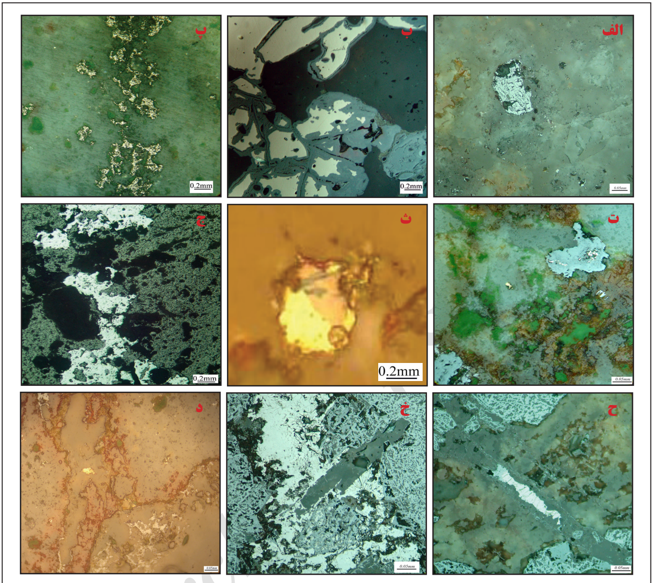
شکل ۶- الف) نمایی میکروسکوپی از مگنتیت ماریتی شده در توده نفوذی همراه با آغشتگی‌های لیمونیتی؛ ب) نمایی از پیریت که از حاشیه‌ها به گوتیت تبدیل شده است؛ پ) تبدیل پیریت به هیدروکسیدهای نهان بلورین پیریت با افزایش شدت هوازدگی؛ ت) نمایی میکروسکوپی از کانی کالکوپیریت که از حاشیه به گوتیت تبدیل شده است؛ ث) نمایی میکروسکوپی از همراهی کالکوپیریت، بورنیت، کالکوسیت و مالاکیت در توف سیلیسی و کربناتی شده؛ ج) نمایی میکروسکوپی از پیریت با بافت باقی مانده که به لپیدو کروزیت و گوتیت تبدیل شده است؛ ح و خ) نمایی از رگه‌های پسولوملان همراه با زمینه جاکوپسیت در سنگ‌های آتشفشانی؛ د) نمایی میکروسکوپی از ترکیب مس - قلع - آهن دار در توف ویترو کلاستیک.
