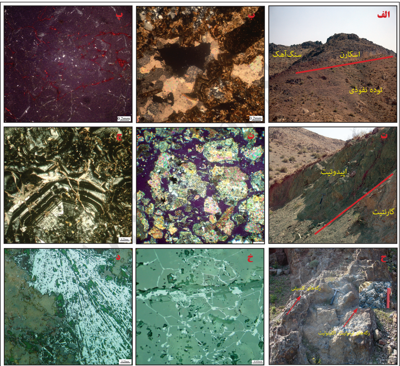
شکل ۹- الف) نمایی از همبندی بین توده نفوذی نیمه‌زرف، اسکارن و آهک (دید به سمت شمال). اسکارن در اثر شار حرارتی توده‌های نفوذی در راستای گسل امتداد لغز با امتداد تقریباً 90° N؛ ب) نمایی میکروسکوپی از یک سنگ آهک دولومیتی که کانه‌زایی آهن را به صورت هم‌رشدی با دولومیت نشان می‌دهد؛ پ) نمایی میکروسکوپی از گارتیت به همراه کانه هماتیت در شکستگی‌ها؛ ت) نمایی از همبندی بین زون اسکارنی پیش‌رونده (حاوی گارتیت) و اسکارن پس‌رونده (حاوی اپیدوت و کمی کلریت) (دید به سمت شمال خاور)؛ ث) نمایی میکروسکوپی از واحد کاملاً اپیدوتی شده؛ ج) نمایی میکروسکوپی از کانی هیدروگروسولار با بافت گرانوبلاستیک که در فضای آن کربنات وجود دارد و گاه رگچه‌های کلسیتی گارتیت را قطع کرده است و تبدیل شدگی گارتیت به اپیدوت نیز دیده می‌شود؛ ح) نمایی از رخنمون واحد اسکارنی همراه با دگرسانی پس‌رونده آمفیبول، کلسیت و اپیدوت و کوارتز (دید به سمت شمال باختر)؛ خ) هماتیت‌هایی که در شکستگی‌های گارتیت جای گرفته‌اند؛ د) هماتیت‌هایی که به صورت شعاعی رشد کرده‌اند.
