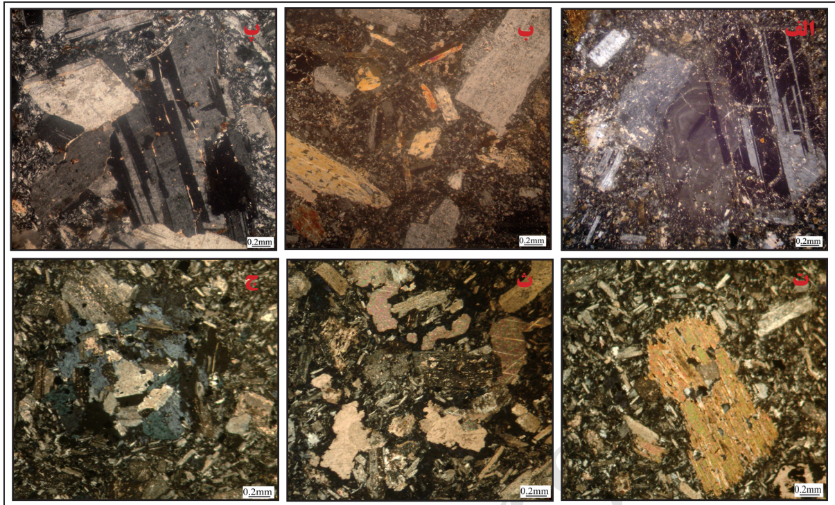
شکل ۴- الف) نمایی میکروسکوپی از منطقه‌بندی پلاژیو کلاز در سنگ با ترکیب مونزودیوریت پورفیری کربناتی و سریستی؛ ب) سنگ با ترکیب مونزودیوریت پورفیری همراه با دگرسانی سریستی که به طور پراکنده به ویژه در پلاژیو کلازها و تبدیل شدگی آمفیبول به ترمولیت- اکتینولیت دیده می‌شود؛ پ) پلاژیو کلاز، فلدسپار آلکالن و کوارتز در سنگ با ترکیب گرانودیوریت پورفیری؛ ت) کانی بیوتیت همراه با ادخال‌هایی از آپاتیت در دایک با ترکیب مونزودیوریت و بافت میکروولیتی- پورفیریتهک؛ ث) حفره‌هایی که با کلسیت پر شده است؛ ج) کانه‌زایی پیریت که با دگرسانی کلریتی همراه شده است (کلیه تصاویر به صورت xpl تهیه شده‌اند).
