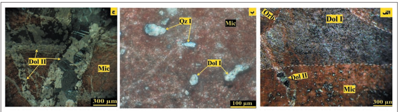
شکل ۱۱- دگرسانی دولومیتی در سنگ‌آهک توده‌ای اربیتولین دار. الف) دولومیت گرمابی (Dol I) جانشین میکروفسیل اربیتولین (Orbitolina Discoidea) شده و رگچه دولومیت (Dol II) زمینه میکربیت و اربیتولین (Orbitolina Discoidea) را قطع کرده است؛ ب) دولومیت گرمابی (Dol I) و کوارتز (Qz I) به صورت پراکنده در متن میکربیت دیده می‌شود؛ ج) رگه- رگچه‌های دولومیت گرمابی (Dol II) شکل دار، زمینه میکربیت را قطع کرده است (مقطع نازک رنگ آمیزی شده در نور XPL).
