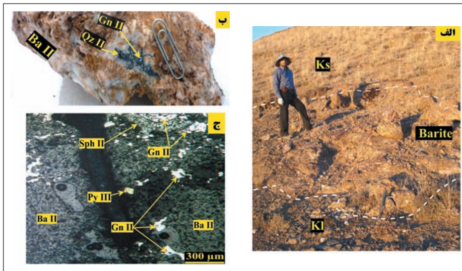
شکل ۹- ساخت و بافت باریت توده‌ای همراه با سولفید در کانسار کوه کلنگه. الف) عدسی باریت توده‌ای در افق اول کانه‌زایی در بخش بالایی Kl و در زیر واحد Ks؛ ب) نمونه دستی کانسنگ توده‌ای باریت، از افق اول کانه‌زایی (شکل الف) دارای باریت توده‌ای (Ba II)، گالن (Gn II) و کوارتز (Qz II)؛ ج) تصویر میکروسکوپی بازتابی، از باریت توده‌ای که در آن اسفالریت (Sph II) جانشین گالن (Gn II) شده است.
