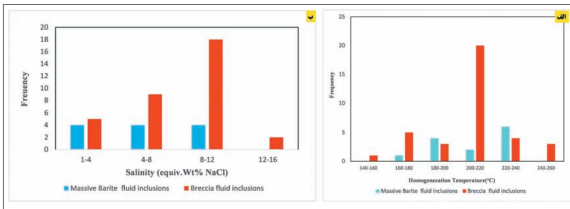
شکل ۱۴- مقایسه توزیع دمای همگن‌شدگی و شوری میان‌بارهای سیال در کانسنگ برشی و باریت توده‌ای؛ الف) نمودار تغییرات دمای همگن‌شدگی میان‌بارهای سیال کانسار کوه کلنگه، که گستره دمایی از ۱۴۰ تا ۲۶۰ درجه سانتی‌گراد دارد؛ ب) نمودار تغییرات شوری میان‌بارهای سیال کانسار مورد مطالعه، که شوری آنها در بازه ۱ تا ۱۶ درصد جای می‌گیرد.
