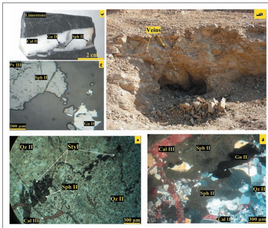
شکل ۸- ساخت و بافت رگه- رگچه‌ای در کانسار کوه کلنگه. الف) رگه - رگچه‌های سیلیسی- کربناتی دارای سولفید، سنگ‌آهک توده‌ای خاکستری اریبتولین دار را قطع کرده است؛ ب) اسفالریت (Sph II) همراه با گالن (Gn II) و رگه رگچه های کلسیت (Cal II) تشکیل دهنده‌های اصلی رگه- رگچه های مرحله اصلی کانه‌زایی کانسار کوه کلنگه هستند؛ ج) تصویر میکروسکوپی از رگه- رگچه‌های سیلیسی- کربناتی دارای اسفالریت (Sph II)، گالن (Gn II) و پیریت (Py III) کانه‌زایی در کانسار کوه کلنگه؛ د) تصویر میکروسکوپی از قطع شدگی رگه- رگچه‌های دارای اسفالریت (Sph II) و گالن (Gn II) توسط رگچه‌های کلسیت (Cal III) یا مرحله تأخیری (مقطع رنگ آمیزی شده در نور XPL)؛ ه) تشکیل اسفالریت (Sph II) در مجاورت استیلولیت (Styl)؛ کل مجموعه توسط کلسیت مرحله سوم (Cal III) قطع شده است (مقطع رنگ آمیزی شده در نور PPL).
