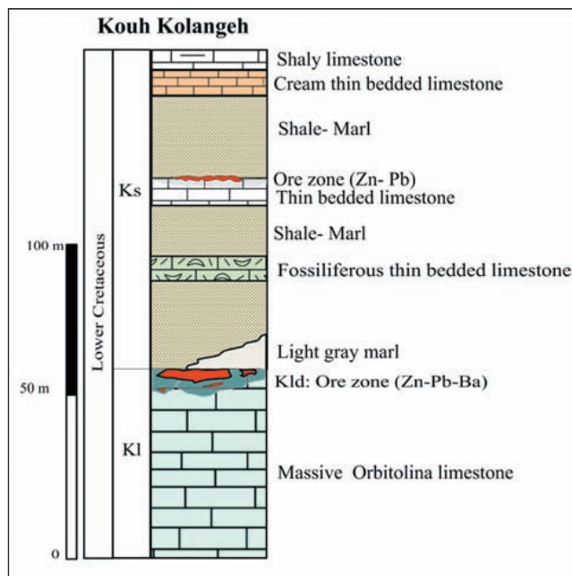
شکل ۴- ستون چینه‌شناسی عمومی کانسار کوه کلنگه و موقعیت جایگاه افق اول کانه‌زایی (K1d) در بخش بالایی سنگ‌آهک سترلایه (K1) و افق دوم کانه‌زایی در سنگ‌آهک نازک‌لایه واحد (Ks).
