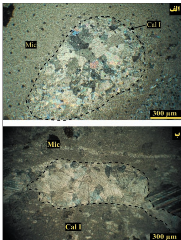
شکل ۵- انواع سیمان کلسیتی در واحد K1 کانسار کوه کلنگه. الف) سیمان کلسیتی Drusy نسل اول، حفرات موجود زمینه میکریت را پر کرده است؛ بلورهای کلسیت (Cal I) از حاشیه به سوی مرکز حفره درشت می‌شوند؛ ب) سیمان کلسیتی Blocky نسل اول در زمینه میکریتی؛ بلورهای کلسیت (Cal I) با مرز مشخص بلوری از متوسط تا درشت و بدون جهت‌یافتگی دیده می‌شوند.
