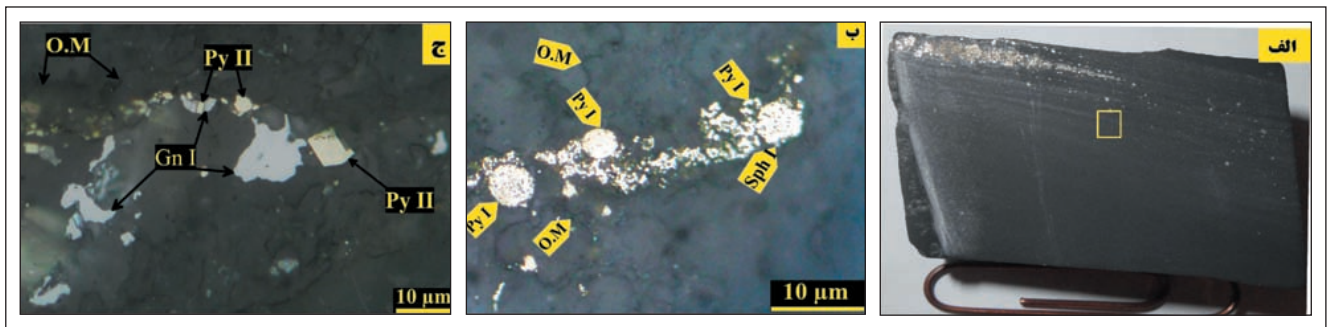
شکل ۱۰- ساخت و بافت لامینه در کانسار روی-سرب- باریت کوه کلنگه. الف) نمونه دستی از سنگ‌آهک میکربیتی غنی از مواد آلی، که لامینه‌های غنی از پیریت (Py I) و اسفالریت (Sph I) با رنگ روشن مشخص است؛ ب) تصویر میکروسکوپی از شکل الف، شامل تجمع پیریت فراموبیدال و اسفالریت (Sph I) در بخش غنی از مواد آلی (O.M)؛ ج) تصویر میکروسکوپی از پیریت‌های خود شکل (Py II) که از تبلور پیریت‌های فراموبیدال (Py I) در طی دیاژنز تشکیل و همراه با گالن نسل اول (Gn I) دیده می‌شود.
