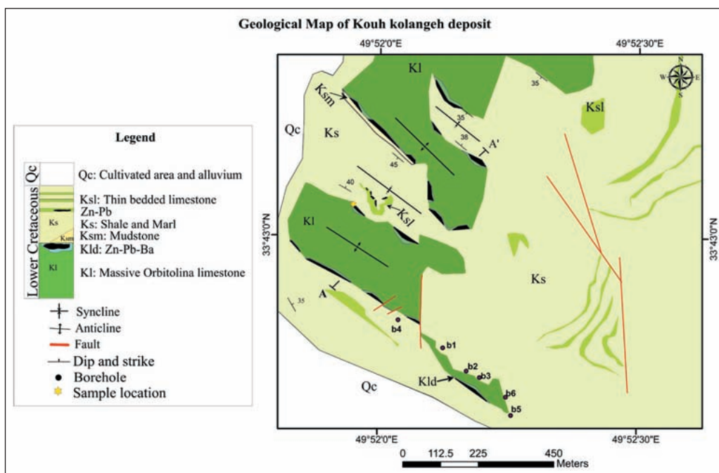
شکل ۲- نقشه زمین‌شناسی کانسار کوه کلنگه و موقعیت کانه‌زایی‌های روی-سرب-باریت در واحدهای چینه‌ای Kl و Ksl.
