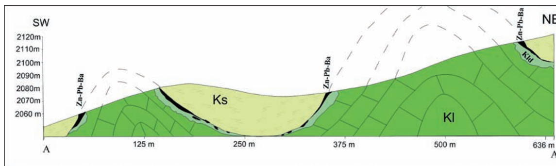
شکل ۳- مقطع زمین‌شناسی (AA) از توالی رسوبی کرتاسه زیرین در منطقه معدنی کوه کلنگه و موقعیت چینه‌ای کانه‌زایی روی-سرب-باریت در آن. چین‌خوردگی‌های بسیار سبب تکرار افق‌های کانه‌زایی شده است (محل مقطع زمین‌شناسی همراه با راهنمای آن روی شکل ۲ مشخص شده است).
