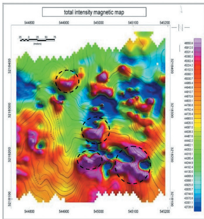
شکل ۳- نقشه شدت کل مغناطیس (مناطق امیدبخش) منطقه فراش کرمان.
