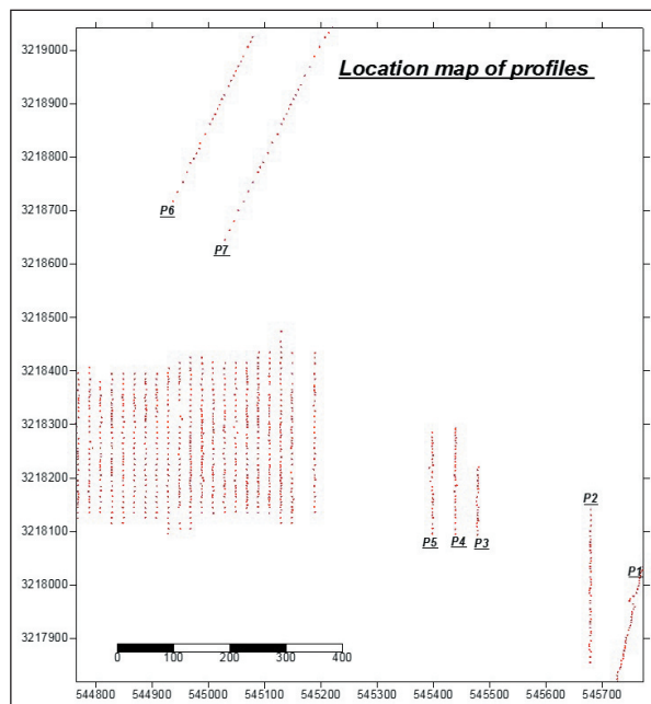
شکل ۴- جانمایی موقعیت نقاط برداشت مغناطیس سنجی.
