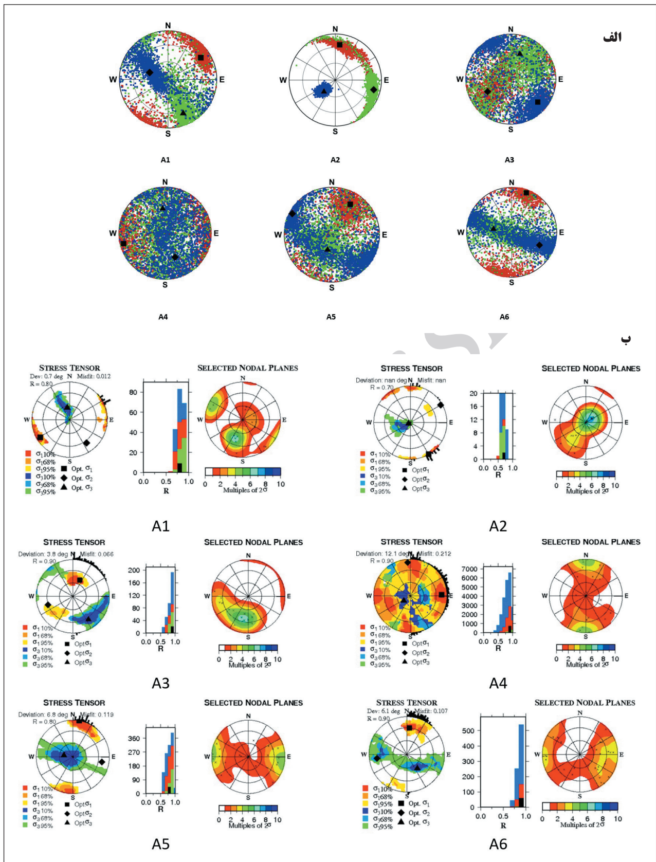
شکل ۳- الف) نتایج وارون‌سازی تنش نشان داده شده در استریونت. نقطه‌های قرمز، سبز و آبی نشان‌دهنده نقاط معرف \sigma_1 ، \sigma_2 و \sigma_3 طی نمونه‌گیری مجدد خود راه‌انداز، از روش Michael (1984) و مربع سیاه، لوزی و مثلث به ترتیب نشان‌دهنده راه حل بهینه برای محورهای تنش مذکور هستند؛ ب) نتیجه وارون‌سازی غیرخطی تنش (Lund and Slunga, 1999) روی داده‌های لغزش گسلی دره دیکسی، به روش زاویه لغزش؛ ب) نتیجه وارون‌سازی غیرخطی تنش (Lund and Slunga, 1999) روی داده‌های لغزش گسلی دره دیکسی، به روش ناپایداری. تانسور تنش بهینه \sigma_1 به شکل مربع، \sigma_2 به شکل لوزی و \sigma_3 به شکل مثلث همراه حدود اطمینان ۱۰٪، ۶۵٪ و ۹۵٪ برای \sigma_1 تیره به روشن از ۱٪ تا ۹۵٪ و \sigma_3 روشن به تیره ناپایداری. بافت‌نمای (هیستوگرام) سیاه پیرامونی جهت فشردگی افقی بیشینه تانسورها را در محدوده اطمینان ۹۵٪ نشان می‌دهد.
