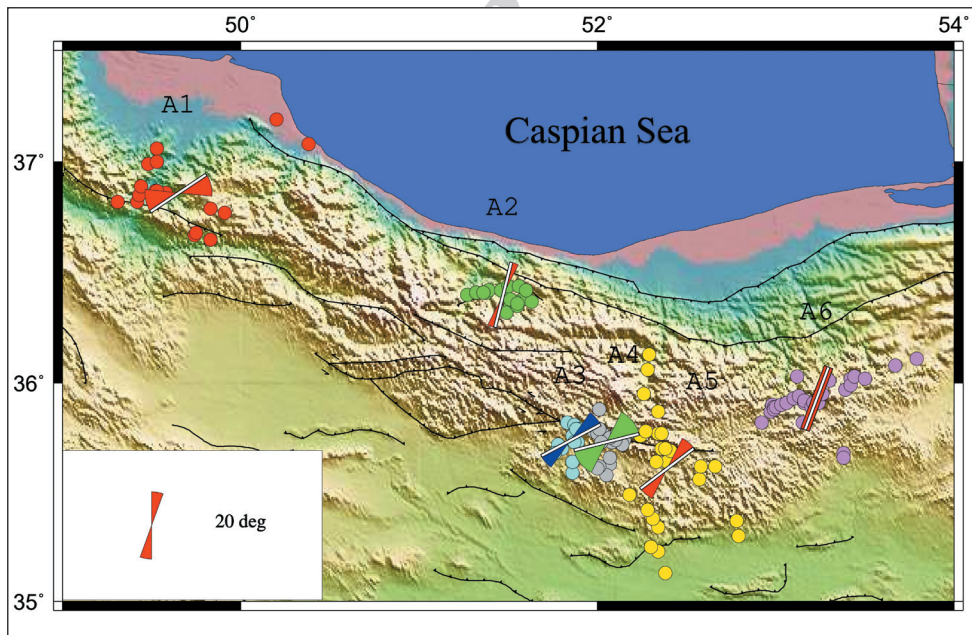
شکل ۶- اختلاف زاویه‌ای بین راستای تنش افقی و محورهای فشارشی آهنگ کرنش. راستای تنش با میله سفید مشخص شده است. در این شکل اختلاف زاویه‌ای میان راستای اصلی تنش و کرنش در مرکز و شمال باختری البرز مرکزی به دلیل چیرگی پدیده افراز دگرشکلی بزرگ‌تر است.
