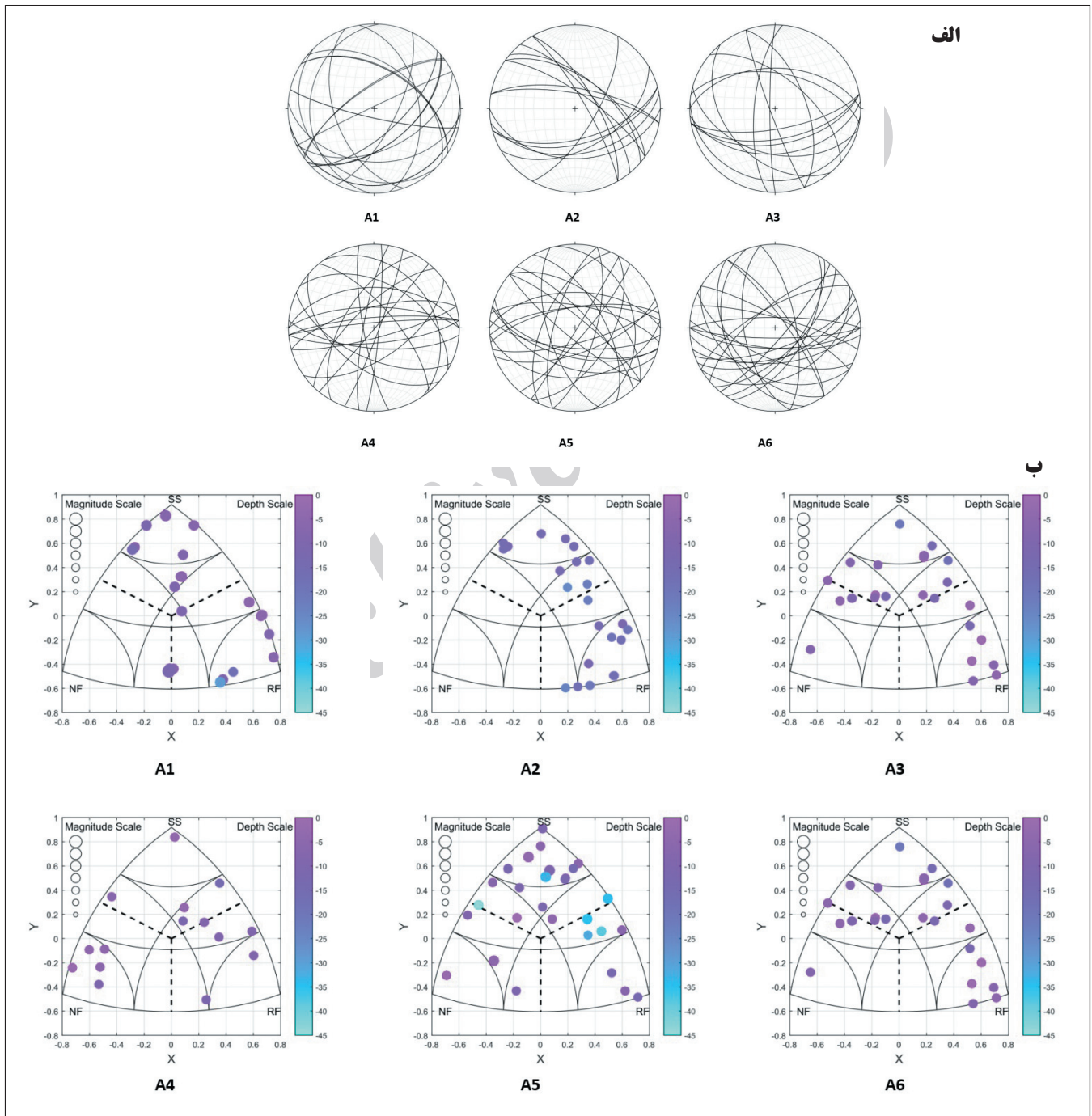
شکل ۲-الف) شیب و امتداد صفحات گسلی به دست آمده از سازوکارهای کانونی زمین‌لرزه‌ها در هر گروه از داده‌ها (ب) طرح مثلثی کیگان سازوکار کانونی زمین‌لرزه‌ها، اندازه دایره‌ها به عنوان بزرگی (از ۱ تا ۷) و عمق توسط مقیاس رنگی نشان داده شده.
