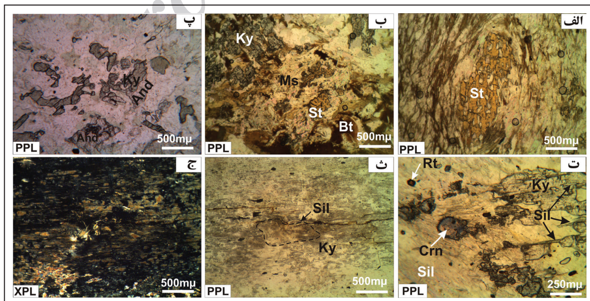
شکل ۵- مقاطع میکروسکوپی شیست‌های منطقه گشت رودخان: الف) پورفیروبلاست استارولیت با بافت پویی کیلیتیک؛ ب) تجزیه استارولیت به میکای سفید در نمونه کیانیت- استارولیت شیست؛ پ) تبدیل آندالوزیت به کیانیت؛ ت) تشکیل منشورهای سیلیمانیت روی کیانیت. کروندوم نیز احتمالاً محصول تجزیه کیانیت است؛ ث) هسته‌بندی فیبرولیت روی کیانیت؛ ج) تصویر ث در نور پلاریزه متقاطع.
