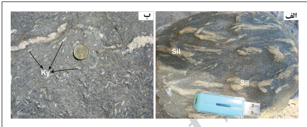
شکل ۲- الف) نمونه ماکروسکوپی سیلیمانیت‌شیت با پورفایرولاست‌های درشت سیلیمانیت؛ ب) نمونه کیانیت‌شیت با پورفایرولاست کیانیت و حالت چین‌خورده.
