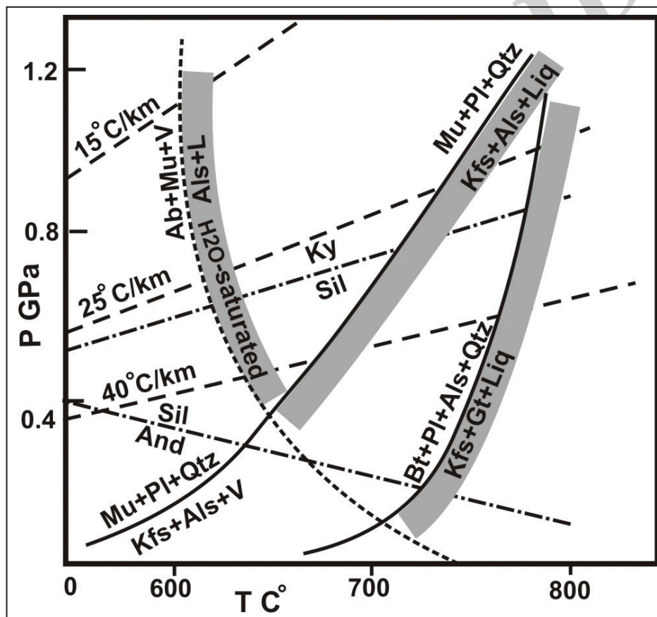
شکل ۸- شبکه پتروژنتیک ساده از متاپلیت‌های درجه بالا (Vielzeuf and Holloway, 1988; Clarke, 1992). سه نوع گرادیان زمین‌گرمایی، واکنش‌های آب‌زدایی مسکوویت و بیوتیت و سالیدوس گرانیته آبدار در این شبکه پتروژنتیک نمایش داده شده است. موقعیت‌های انجام ذوب‌بخشی، به‌صورت باند خاکستری هستند.
