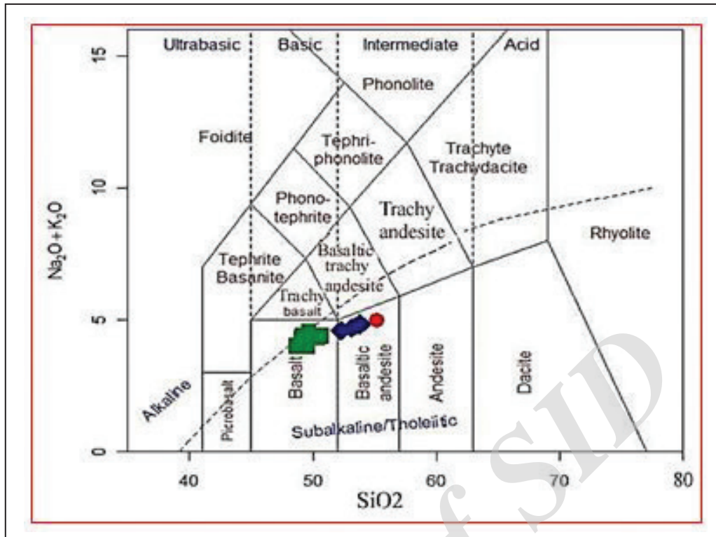
شکل ۱۳- موقعیت نمونه‌های سنگی آتشفشان کوه زا بزرگ، کوه زا کوچک و کوه سُم در نمودار رده‌بندی ژئوشیمیایی (Le Bas et al., 1986)؛ تمامی نمونه‌ها، در محدوده بازالت تا آندزیت بازالت و محدوده ساب آلكالین قرار می‌گیرند.
