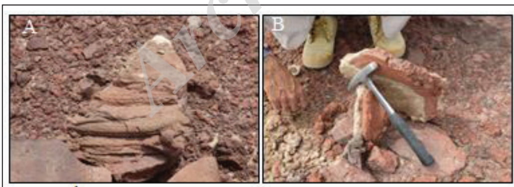
شکل ۳- A) اشکال (A) طنابی و (B) صاف در گدازه‌های بازالتی کوه زا بزرگ.
