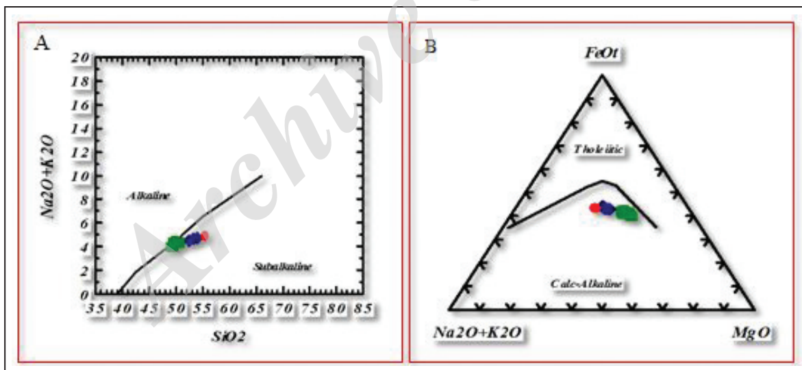
شکل ۱۴- (A) موقعیت نمونه‌های مورد مطالعه در محدوده سری ساب آلكالین، نمودار پایه از (Irvine and Baragar (1971)؛ (B) موقعیت نمونه‌های مورد مطالعه در محدوده سری کالک آلكالین در نمودار پایه (Irvine and Baragar (1971).
