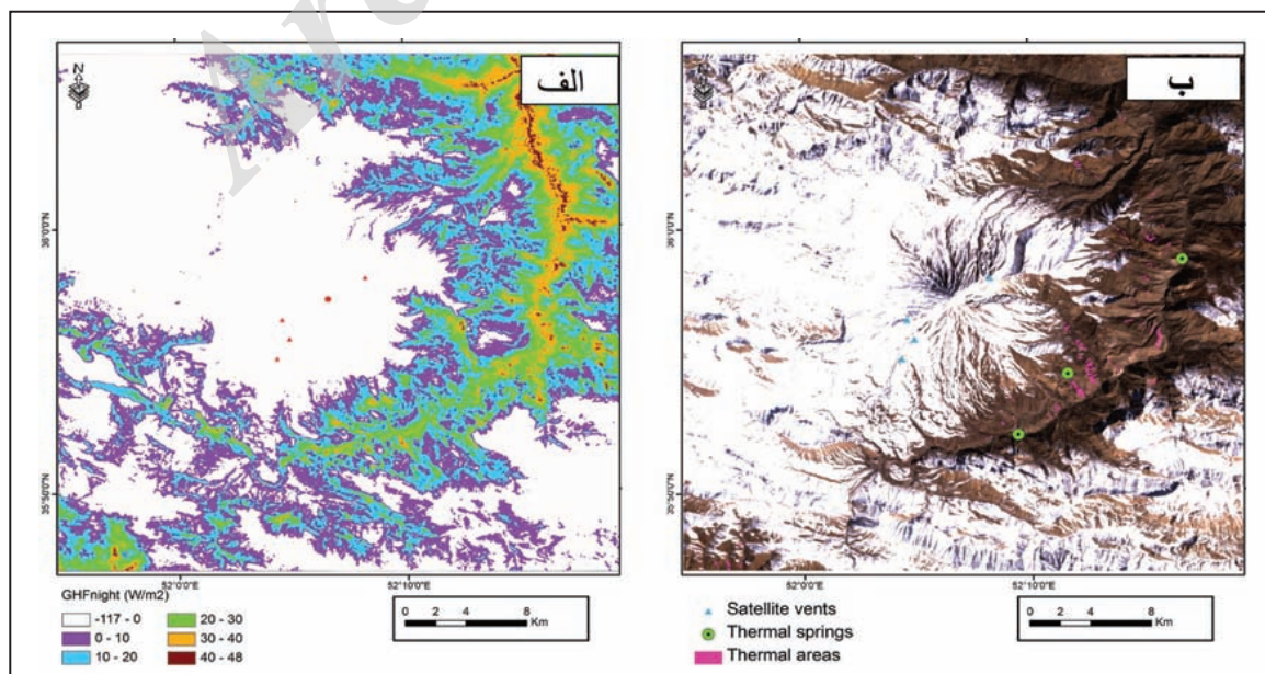
شکل ۴- الف) نقشه GHF به دست آمده از تصویر شب در منطقه آتشفشان دماوند؛ ب) تصویر با ترکیب باندی واقعی ۳۲۱ به دست آمده از تصویر زمستان منطقه آتشفشان دماوند که مناطق با ناهنجاری حرارتی بر روی آن نمایش داده شده است.
