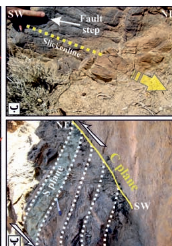
شکل ۱۴- مشخصات و ویژگی‌های گسل X: الف) نمای از گسل X در بازدید صحرائی و تصویر استریوگرافیک گسل؛ ب) موقعیت خشل‌لغز بر روی صفحه گسل؛ پ) صفحات C-S مشاهده شده در امتداد صفحه این گسل نشان‌دهنده سازوکار چپ‌بر گسل.
