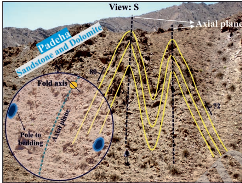
شکل ۷- موقعیت چین H3 در بازدید صحرایی، لایه‌بندی و صفحه محوری و نمودار کانتوری قطب‌های لایه‌بندی در تصویر استریوگرافیک.
