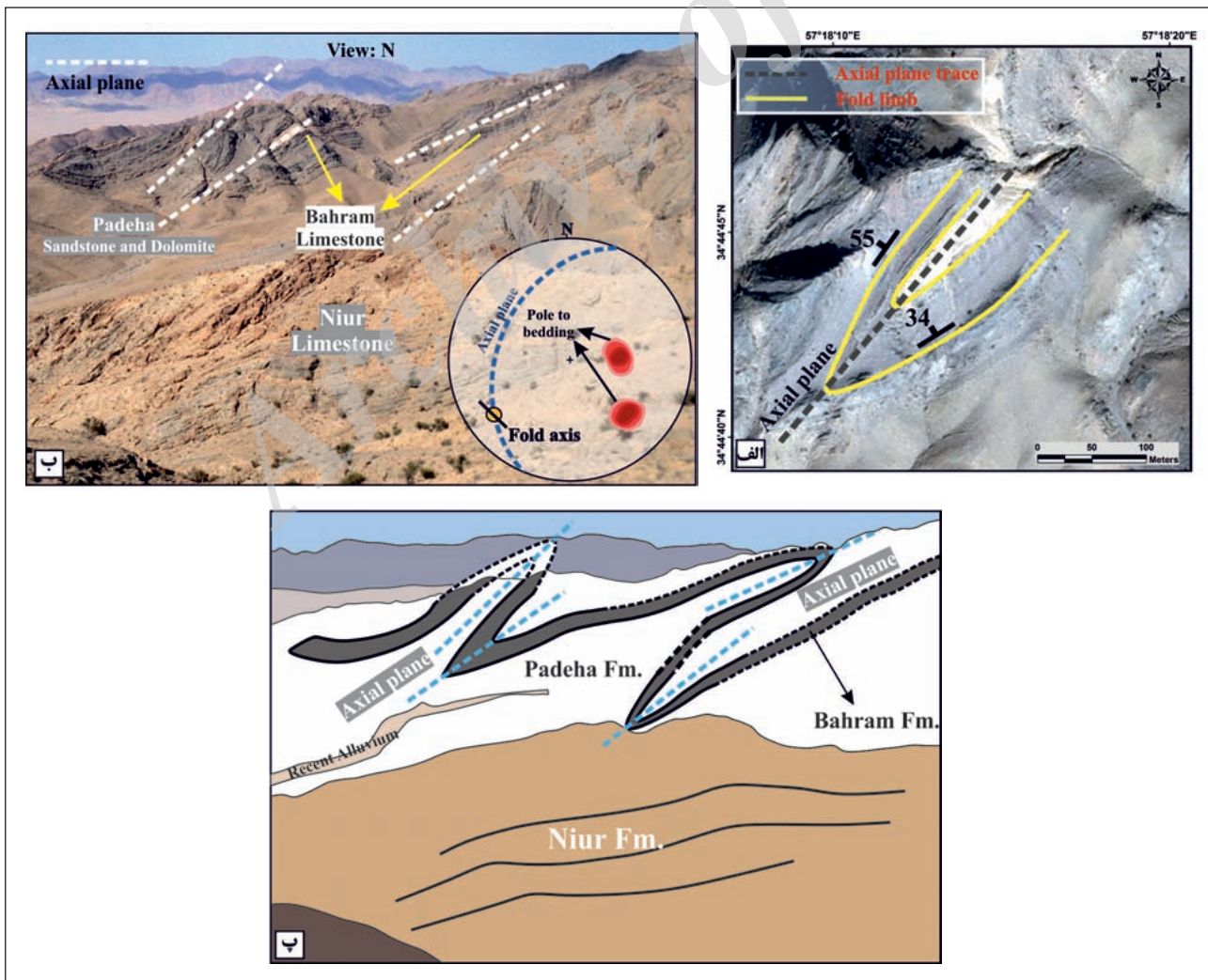
شکل ۸- مشخصات و ویژگی‌های چین H4 (الف) موقعیت چین در تصویر ماهواره‌ای SAS planet به همراه لایه‌بندی و سطح محوری؛ (ب) موقعیت چین H4 در بازدید صحرایی از ازبک کوه، قطب‌های لایه‌بندی و صفحه محوری چین در تصویر استریوگرافیک؛ (پ) مدل شمانتیک و شکل گویا شده چین H4.
