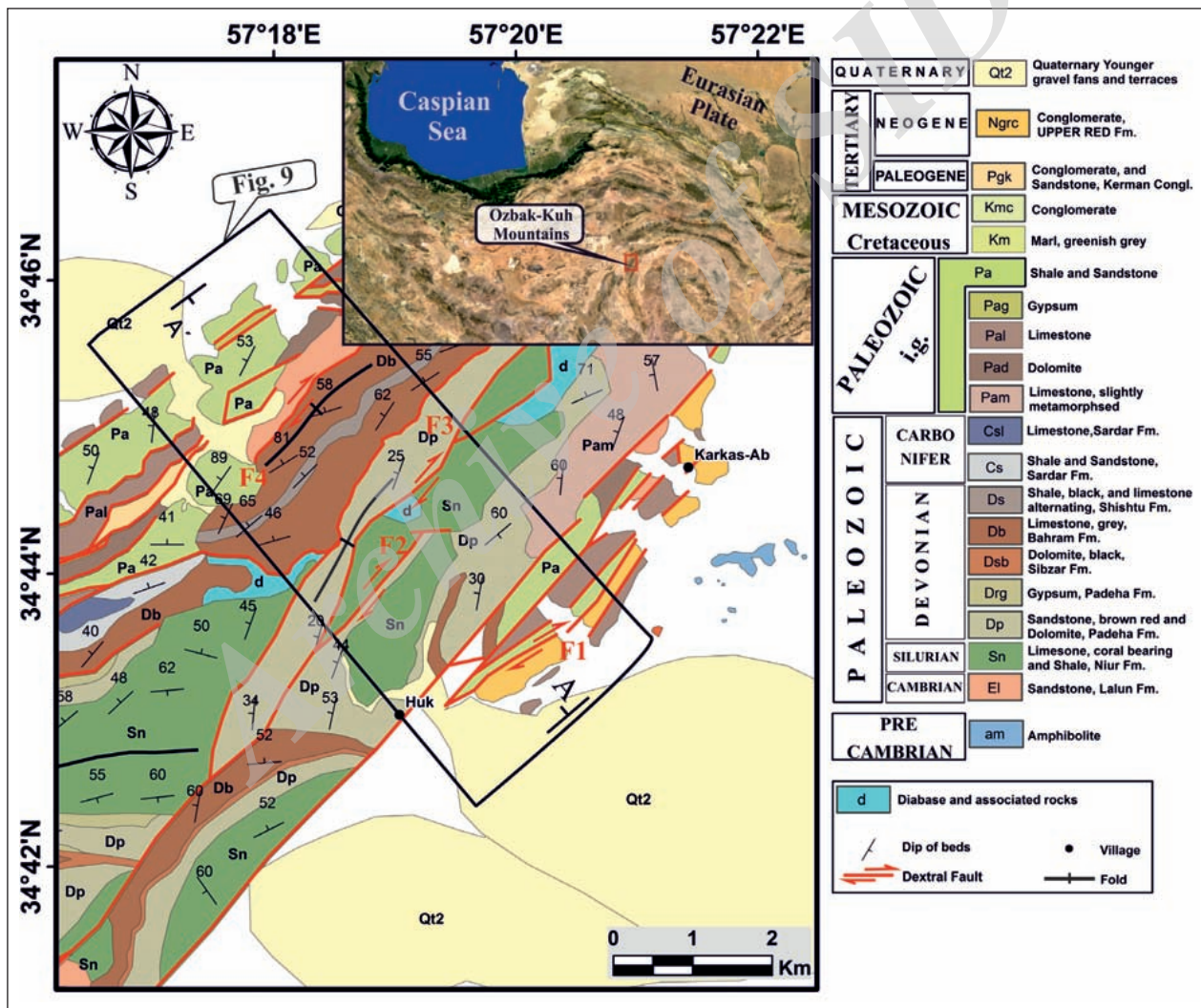
شکل ۲- نقشه زمین‌شناسی ۱:۵۰,۰۰۰ شمال ازبککوه و محل برش ساختاری در آن (واحدهای چینه‌شناسی برگرفته از Ruttner et al., 1968).
