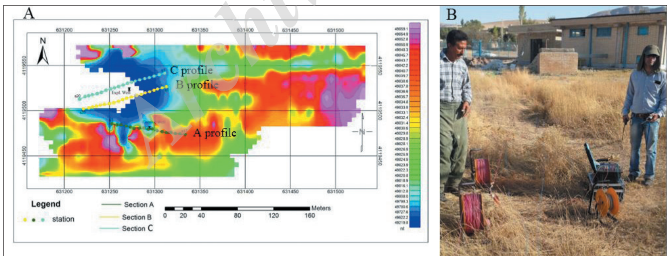
شکل ۷- برداشت‌های مقاومت ویژه الکتریکی. (A) موقعیت پروفیل‌ها و ایستگاه‌های توموگرافی الکتریکی دوبعدی روی نقشه شدت میدان کل؛ (B) تجهیزات برداشت میدانی ژئوالکتریک در داخل محدوده حصار فلزی.
