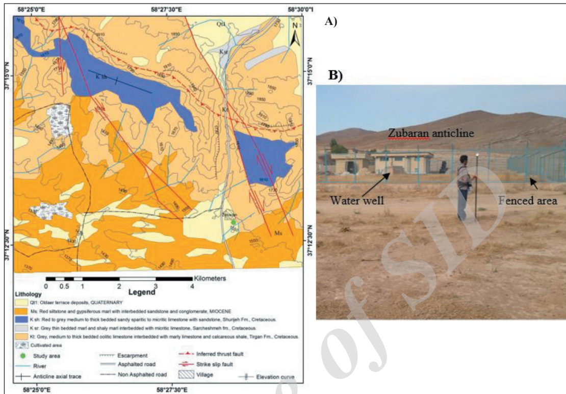
شکل ۲- زمین‌شناسی و تصویر سایت مورد مطالعه. (A) نقشه زمین‌شناسی و توپوگرافی ۱/۱۰۰۰۰۰ منطقه؛ (B) برداشت مغناطیس‌سنجی به عنوان فاز اولیه مطالعات. موقعیت چاه موجود و رخنمون سازند تیرگان (تاقدیس زوباران) در شکل مشخص شده است.
