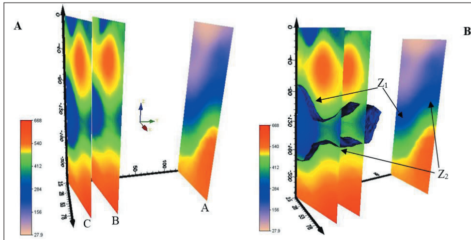
شکل ۹- نمودار فیزیکی یک نمای سه بعدی از مقاطع مقاومت ویژه را نمایش می دهد. زون های رسانا ( Z_1 و Z_2 ) در قسمت های میانی مقاطع مرتبط با نواحی کارستی هستند.
