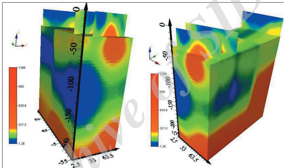
شکل ۱۰- بلوک سه بعدی مدل مقاومت ویژه الکتریکی محدوده مورد مطالعه. فلش سبز رنگ جهت جنوب و بردار قرمز جهت غرب را نشان می دهد. سنگ آهک متراکم با رنگ های قرمز تا سبز نشان داده شده است. رنگ آبی زون های کارستی هستند.
