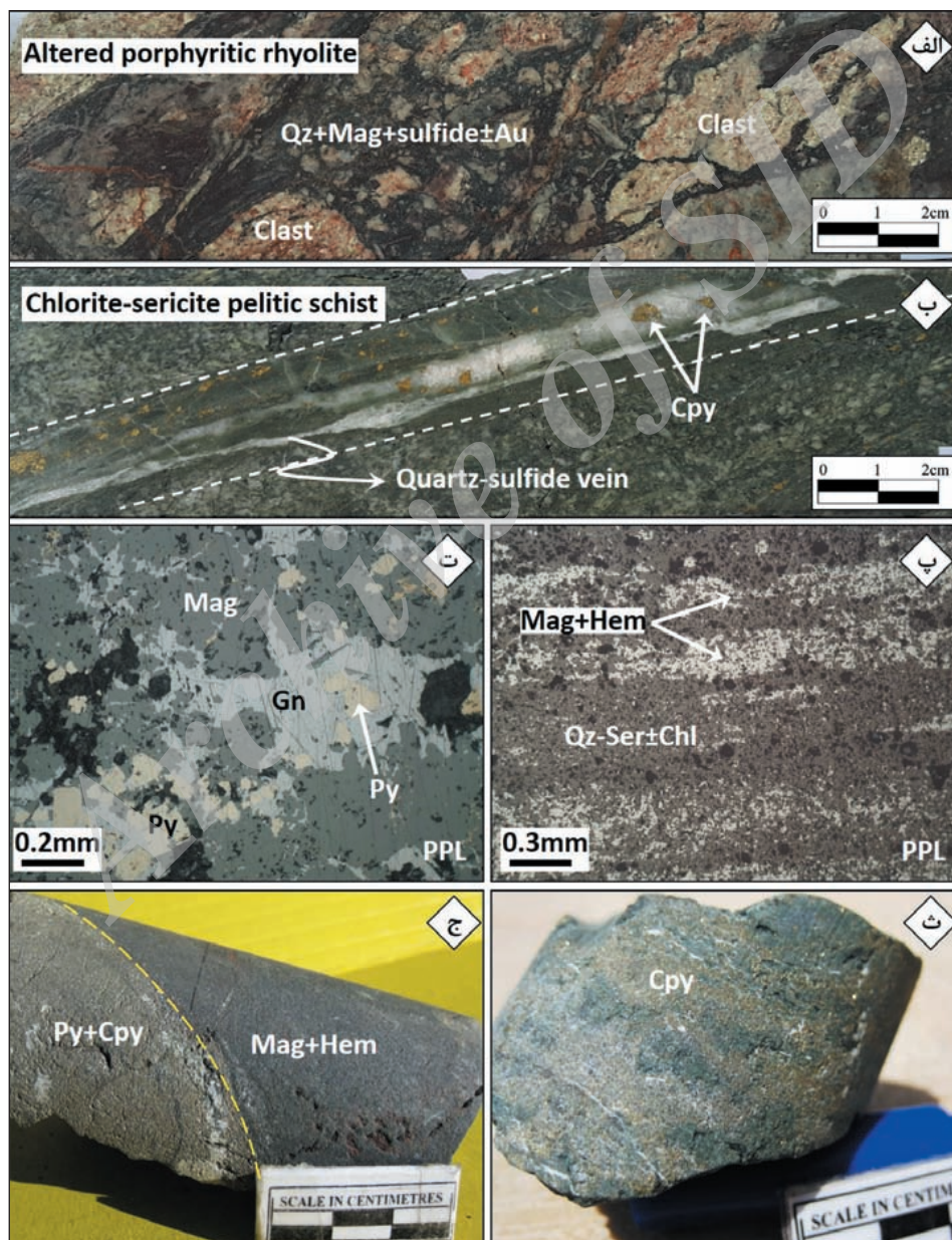
شکل ۵- تصاویر بافت و ساخت کانه‌زایی. الف) کانی‌سازی برشی کوارتز-مگنتیت-سولفید در میزبان ریولیت پورفیری؛ ب) رگه کوارتز-سولفید در میزبان کلریت-سریسیت پلئیتیک شیسست؛ پ) تصویر میکروسکوپی بازتابی از باندهای متناوب مگنتیت-هماتیت در میزبان باطله کوارتز-سریسیت \pm کلریت؛ ت) تصویر میکروسکوپی بازتابی از پاراژنز کانی‌های سولفیدی گالن و پیریت همراه با مگنتیت؛ ث) کانی‌سازی رگه-رگچه‌ای کالکوپیریت در میزبان کلریت شیسست؛ ج) کانی‌سازی سولفید توده‌ای در مجاورت کانسنگ مگنتیت-هماتیت. حروف اختصاری کانی‌ها از Whitney and Evans (2010) شامل Hem=هماتیت، Chl=کلریت، Ser=سریسیت، Py=پیریت، Cpy=کالکوپیریت، Mag=مگنتیت، Gn=گالن، Qz=کوارتز.
