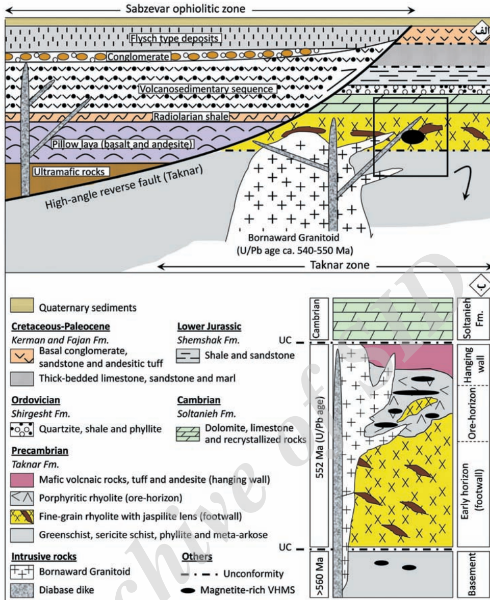
شکل ۱- الف) تصویر شماتیک از واحدهای چینه‌شناسی- ساختمانی زون‌های تکنار و افیولیت سبزوآر (با مقیاس فرضی)؛ ب) ستون چینه‌شناسی واحدهای سنگی شمال کبودان. برگرفته از برگه ۱:۱۰۰۰۰۰ بردسکن (شهرابی و همکاران، ۱۳۸۵) و نقشه زمین‌شناسی ۱:۲۵۰۰۰ کبودان (صفری، ۱۳۸۸).
