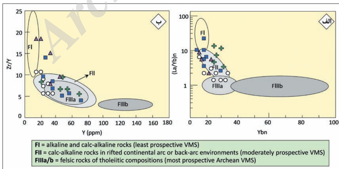
شکل ۹- نمودارهای دوتایی الف) (La/Yb)_n در مقابل Yb_n ؛ ب) نسبت Zr/Y در مقابل Y (به منظور تفکیک سنگ‌های آتشفشانی فلسیک کانه‌دار (prospective) و عقیم (barren)). محدوده‌ها از Leshner et al. (1986) و با تغییرات از Hart et al. (2004). در نمودار الف مقادیر نسبت به کندریت به‌نچار شده‌اند (Nakamura, 1974). همان‌طور که مشاهده می‌شود سنگ‌های منطقه اغلب در گستره‌های سنگی FII (تا حدودی کانه‌دار) و FIIIa (اغلب کانه‌دار) قرار می‌گیرند.
