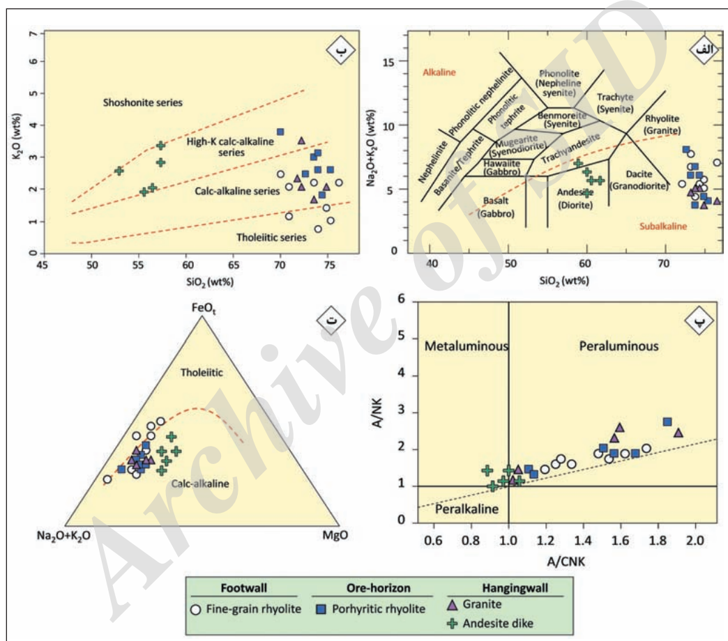
شکل ۶- نمودارهای ژئوشیمی عناصر اصلی در واحدهای سنگی آذرین منطقه کبودان. الف) نمودار دوتایی SiO_2 در مقابل عناصر قلیایی (Le Bas et al., 1986)؛ ب) تعیین میزان آلکالینته سنگ‌ها با استفاده از نمودار دوتایی SiO_2 در مقابل K_2O (Le Maitre et al., 1989)؛ پ) گستره مت‌آلومین تا پرآلومین سنگ‌های منطقه در نمودار دوتایی A/CNK در مقابل A/NK (Maniar and Piccoli, 1989)؛ ت) روند کالک‌آلکان تا کمی تولیتی در نمودار سه‌تایی AFM (Irvine and Baragar, 1971).
