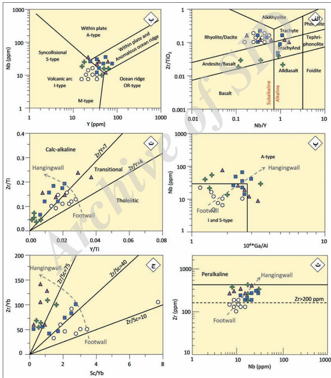
شکل ۷- نمودارهای ژئوشیمی عناصر کمیاب غیرمتحرک در واحدهای سنگی منطقه کیودان. الف) نمودار دوتایی نسبت Zr/TiO 2 در مقابل Nb/Y (Pearce, 1996)؛ ب) تعیین جایگاه زمین‌ساختی در نمودار دوتایی Nb در مقابل Y (Pearce et al., 1984)؛ پ) تعیین تیپ سنگ‌ها در نمودار دوتایی Nb در مقابل Ga/Al (Whalen et al., 1987)؛ ت) تعیین سری‌های ماگمایی و نسبت Zr/Y سنگ‌ها در نمودار دوتایی Zr/Ti در مقابل Y/Ti (Lentz, 1998 and 1999)؛ ث) بررسی محتوای HFSE واحدهای سنگی مختلف در نمودار دوتایی Zr در مقابل Nb (Leat et al., 1986)؛ ج) مقایسه نسبت HFSE به عنصر سازگار (نظیر نسبت Zr/Sc) با استفاده از نمودار دوتایی Zr/Yb در مقابل Sc/Yb (Piercy et al., 2001). نمادها مانند شکل ۶.
