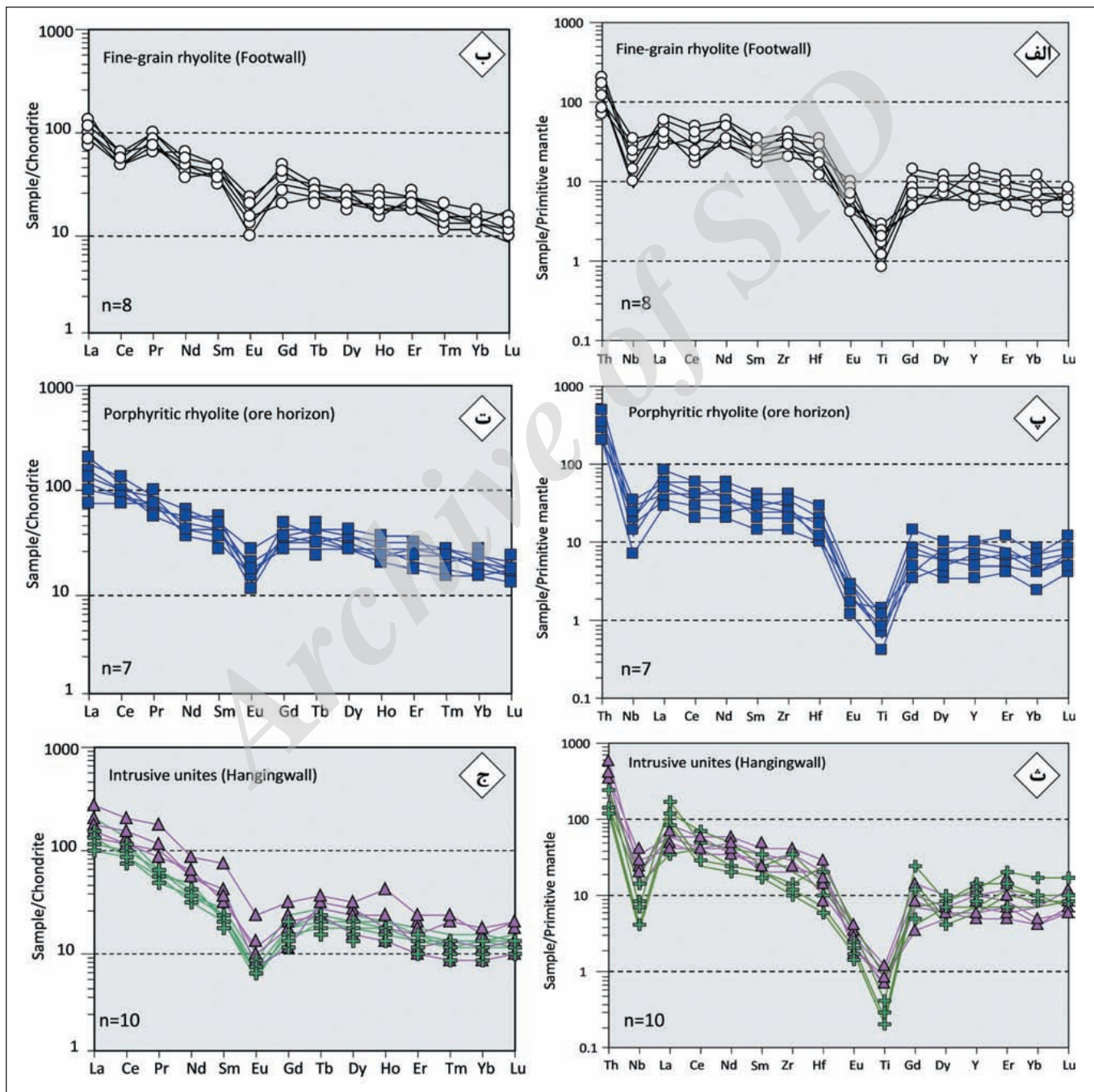
شکل ۸- نمودارهای عنکبوتی بهنجار شده نسبت به گوشته نخستین (Sun and McDonough, 1989) و کندریت (Boynton, 1984) به ترتیب در واحدهای سنگی منطقه شامل الف و ب) ریولیت‌های ریزبلور افق زیرین؛ پ و ت) ریولیت‌های پورفیری افق کانه‌دار؛ ث و ج) آندزیت و گرانیت‌های افق تأخیری. نمادها مانند شکل ۶.
