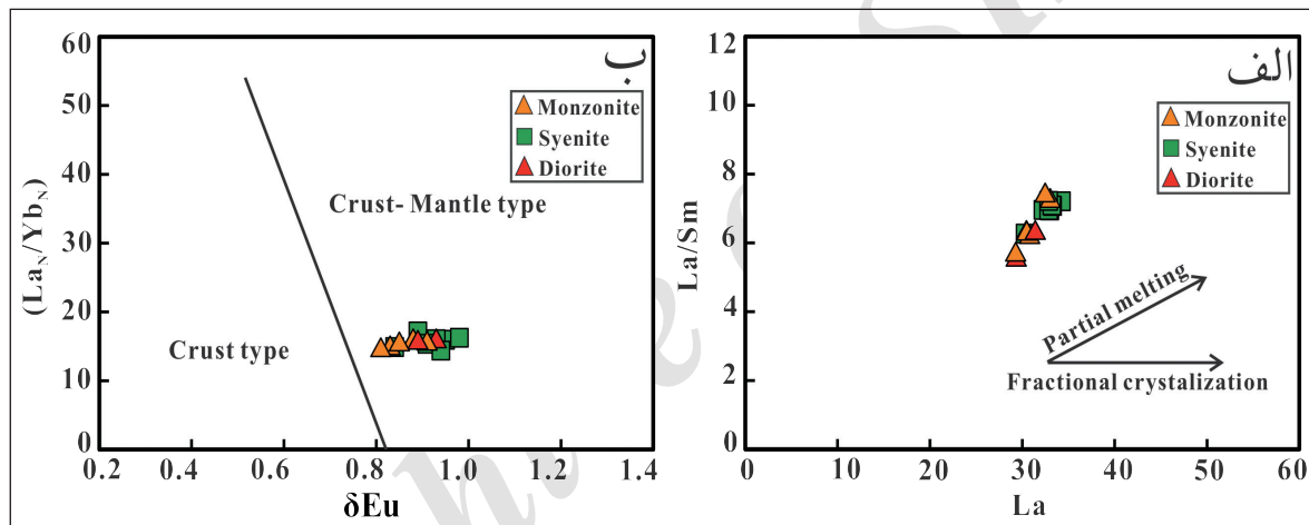
شکل ۹- نمودار La در برابر La/Sm (الف)؛ نمودار δEu در برابر (LaN/YbN) (ب) (Zhang et al., 2014)؛ نمودار La در برابر La/Sm (الف)؛ نمودار δEu در برابر (LaN/YbN) (ب) (Li et al., 2011).
