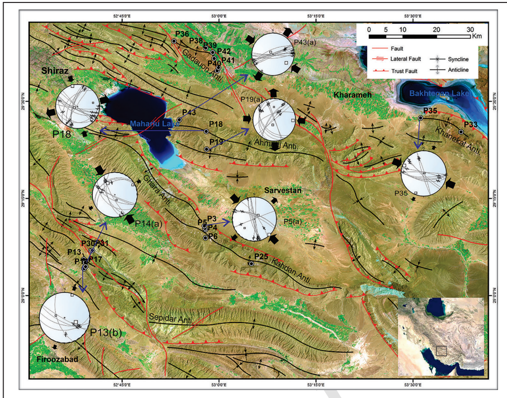
شکل ۸- استریوپلات‌های دسته‌های گسلی امتدادلغز پس از چرخش که جهت کشش شمال خاور- جنوب باختر را نشان می‌دهند و جایگاه آنها در عکس نقشه ساختاری محدوده مورد بررسی.
