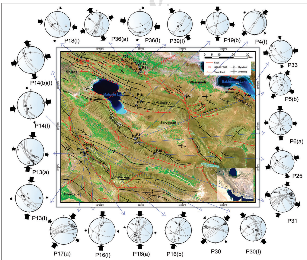
شکل ۹- استریوپلات‌های دسته‌های گسلی رانندگی پس از چرخش و گسل‌های راستالغز که جهت فشارش غالب را نشان می‌دهند و جایگاه آنها در عکس نقشه ساختاری محدوده مورد بررسی.
