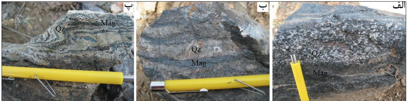
شکل ۶- الف و ب) نمایی نزدیک از کانه‌زایی آهن در رخدادهای معدنی میانجی به‌صورت تناوب نوارهای مگنتیت و کوارتز با ساخت لامینه‌ای؛ پ) چین‌خوردگی در نوارهای مگنتیت و کوارتز (علایم اختصاری کانی‌ها همانند شکل ۳).
