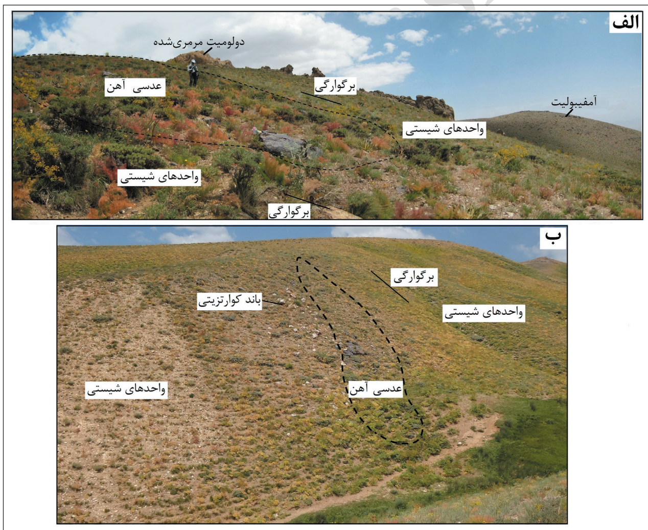
شكل ۵- تصاوير صحرايى از رخنمون ماده معدنى در ميانج. الف) عدسى اصلى آهن هم‌روند با برگوارگى واحدهاى شيبستى (ديد به سوي شمال)؛ ب) عدسى آهن همراه با يك باندهاى كوارتزيتى هم‌روند با برگوارگى واحدهاى شيبستى (ديد به سوي شمال باختر).
