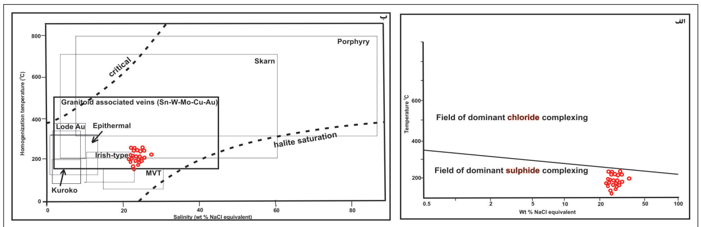
شکل ۱۱-الف) نمودار دمای همگن‌شدگی-شوری سیالات به منظور تعیین کمپلکس (آنیون) مؤثر در حمل عناصر کنسار ساز (Pirajno, 2009) که نقش SO_4^{2-} و یا HS^- را در مس زرنده برجسته می‌سازد؛ ب) نمودار تعیین تیپ کانه‌زایی براساس شوری و دمای همگن‌شدگی (Wilkinson, 2001) که مس زرنده در موقعیت کانی‌سازی‌های رگه‌ای مرتبط با گرانیتوئیدها قرار می‌گیرد.
