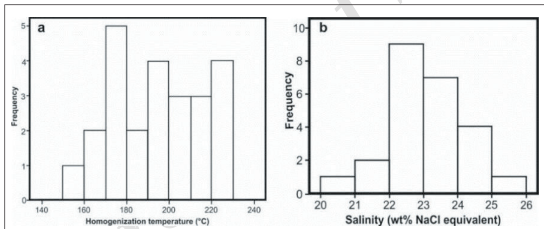
شکل ۸- نمودار ستونی درجه حرارت همگن‌شدگی (a) و شوری (b) میانبارهای سیال منطقه زرنده نسبت به فراوانی آنها.
