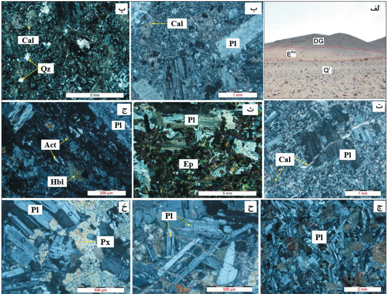
شکل ۴- تصاویر صحرایی و میکروسکوپی از سنگ‌های آذرین منطقه زرننده. الف) نمای از همبری سنگ‌های دیوریت- گابرو (DG)، ریوداسیت ( E^{Rd} ) و آبرفت‌های کواترنری ( Q' ) با دید به سمت جنوب منطقه؛ ب) تصویر میکروسکوپی داسیت با بافت پورفیری با زمینه میکرو کریستالین؛ پ) تصویر میکروسکوپی از ریوداسیت با بافت پورفیری؛ ت) تصویر میکروسکوپی نمونه‌ای از واحد آندزیتی؛ ث) تصویر میکروسکوپی دیوریت که اپیدوتی شده؛ ج) تصویر میکروسکوپی دیوریت حاوی اکتینولیت‌های ریز سوزنی و هورنبلند؛ چ) تصویر میکروسکوپی از گابردیوریت؛ ح) بافت اینترسرتال در گابرو دیوریت؛ خ) بافت افیتیک در گابرو دیوریت (Pl: پلاژیو کلاز، Cal: کلسیت، Qz: کوارتز، Ep: اپیدوت، Act: اکتینولیت، Hbl: هورنبلند، Px: پیروکسن).
