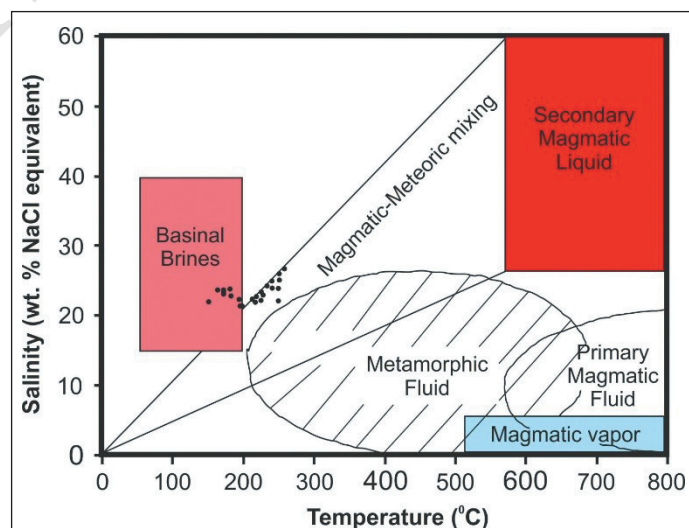
شکل ۹- نمودار درجه حرارت- شوری برای سیالات با منشأهای متفاوت (Beane, 1983). که نمونه‌های زرنده در محدوده اختلاط آب‌های ماگمایی - جوی قرار گرفته‌اند.
