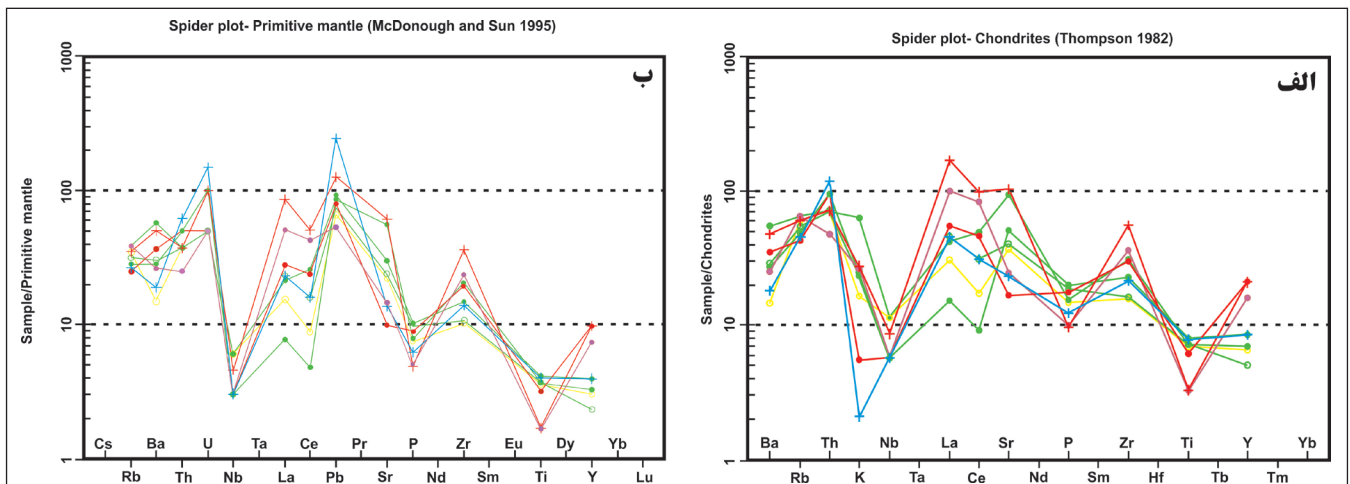
شکل ۶- نمودارهای عنکبوتی بهنجار شده سنگ‌های آذرین زرنديه نسبت به: الف) کندریت (Thompson, 1982)؛ ب) گوشته اولیه (McDonough and Sun, 1995).
