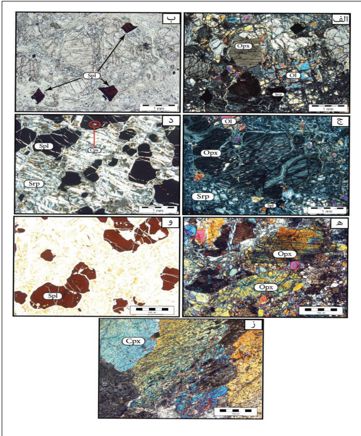
شکل ۳- الف) حضور کانی‌های الیوین، ارتوپیروکسن و اسپینل در هارزبورژیت‌های منطقه مورد مطالعه؛ ب) اسپینل‌های قهوه‌ای رنگ با حواشی تیره همراه با الیوین و ارتوپیروکسن‌های درشت در هارزبورژیت (نور ppl)؛ ج) تیغه‌های اکسلوشن کلینوپیروکسن در ارتوپیروکسن‌های درشت بلور در هارزبورژیت‌های مورد مطالعه؛ د) دونیت متشکل از اولیوین، اسپینل‌های ریز تا درشت تیره رنگ با ادخال کلینوپیروکسن در زمینه اولیوین‌های سرپانتینی شده؛ ه) خمیدگی رخ‌ها و حالت کینک‌بند در بلورهای ارتوپیروکسن هارزبورژیت؛ و) بلورهای قهوه‌ای رنگ و حالت کرمی‌شکل اسپینل در دونیت؛ ز) بلورهای درشت کلینوپیروکسن در دایک‌های کلینوپیروکسنیت.
