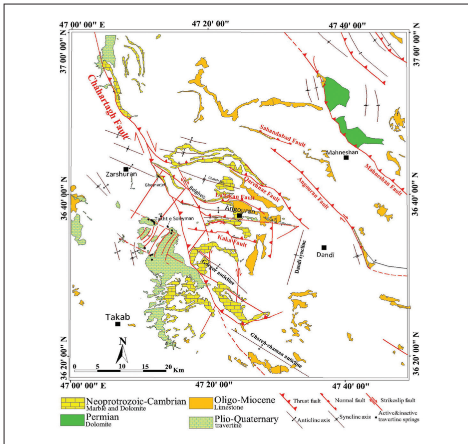
شکل ۳- گسترش کربنات‌ها در منطقه مورد مطالعه، که شامل کربنات‌های جانگوتاران، دولومیت‌های پرمین، آهک‌های الگومیوسن و
