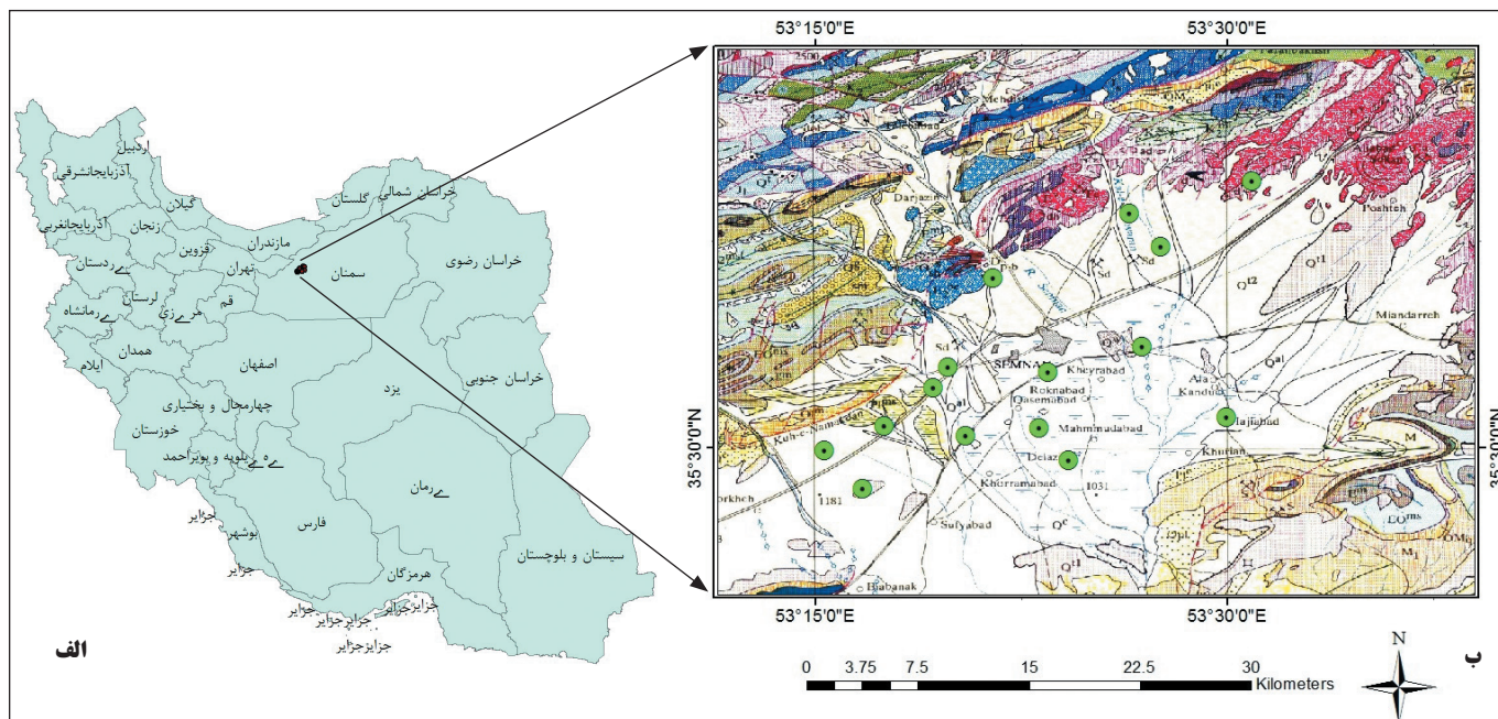
شکل ۲- الف) نمایش موقعیت جغرافیایی محدوده مطالعاتی در استان سمنان؛ ب) نقشه زمین‌شناسی تهیه شده از منطقه با اقتباس از آقائباتی و حامدی (۱۳۷۳) (نقاط سبز رنگ جانمایی چاه‌های مشاهده‌ای را نمایش می‌دهد).
