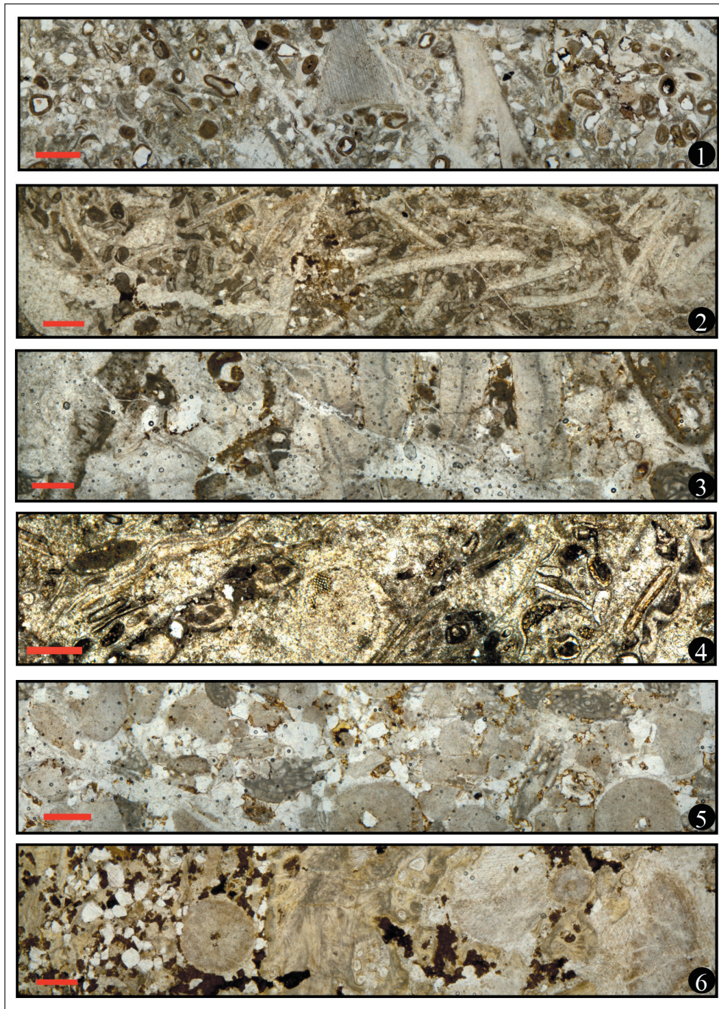
شکل ۵- میکرو فاسیس افق های مرجانی مورد مطالعه. (۱) پکستون بیوکلستی، محیط لاگون؛ (۲ و ۳) پکستون بیوکلستی، محیط دریای باز؛ (۴) گرینستون آئیدی کرینویددار، محیط سد؛ (۵) پکستون بیوکلستی، محیط لاگون؛ (۶) پکستون بیوکلستی، محیط لاگون به سمت سد (مقیاس ۳ میلی متر).
