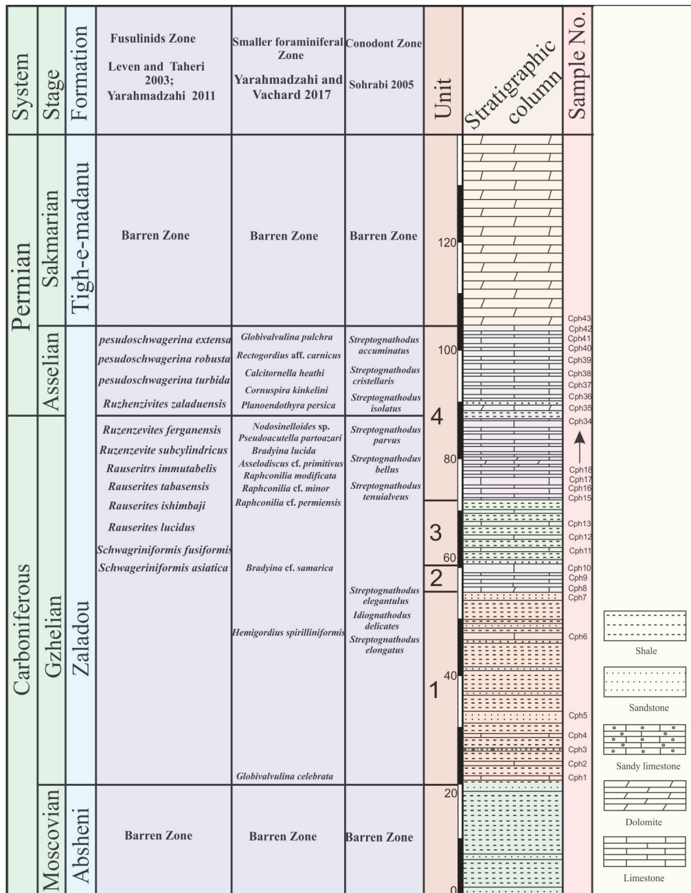
شکل ۲- ستون چینه‌نگاری سنگی برش زلدو. www.SID.ir
