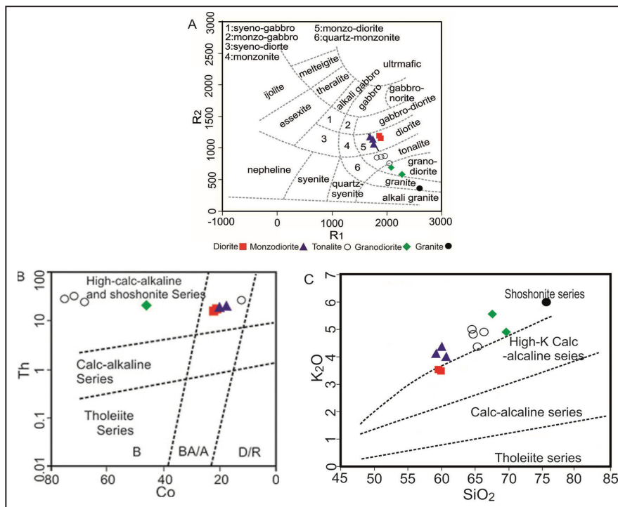
شکل ۳- A) نمودار رده شیمیایی بر حسب R1 در مقابل R2 (De la Roche et al., 1980)؛ B) نمودارهای Co در مقابل Th (Hasti et al., 2007) و SiO_2 در مقابل K_2O (Peccerillo and Taylor, 1976) جهت تعیین سری ماگمایی نمونه‌های مورد بررسی.
