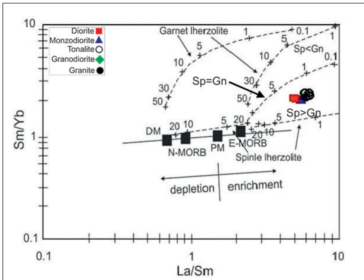
شکل ۱۱- نمودار در مقابل La/Sm جهت تشخیص کانی‌شناسی سنگ منشأ و نیز تخمین درصد ذوب بخشی برای ایجاد ماگمای والد سنگ‌های گرانیتوئیدی محدوده کودکان (O 160 +Opx 20 +Cpx 10 +Gn 10 ): Garnet lherzolite (O 160 +Opx 20 +Cpx 10 +Gn 10 ): Spinel lherzolite (O 160 +Opx 20 +Cpx 10 +Gn 10 ): DM: گوشته تهی شده (بر اساس مقدار عنوان شده توسط McKenzie and O'Nions, 1991)؛ PM: گوشته اولیه یا غنی شده، N-MORB: بازالت پشته میان اقیانوسی نرمال و E-MORB: بازالت پشته میان اقیانوسی غنی شده (بر اساس مقادیر عنوان شده توسط Sun and Mc Donough (1989)).
