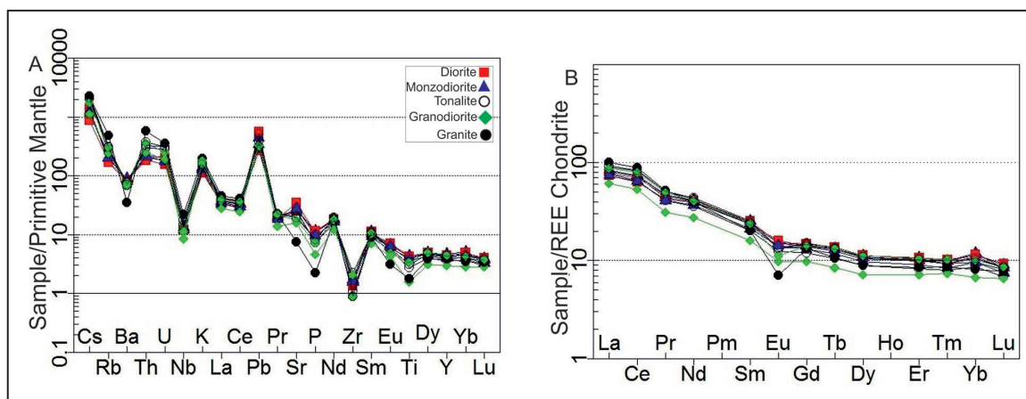
شکل ۶- الگوی عناصر جزئی بهنجار شده بر اساس گوشته اولیه برای نمونه‌های گرانیتوئیدی محدوده مورد مطالعه (Sun and McDonough, 1989)؛ (B) الگوی عناصر نادر خاکی بهنجار شده بر اساس ترکیب کندریت برای نمونه‌های گرانیتوئیدی محدوده مورد مطالعه (Boynton, 1984).
