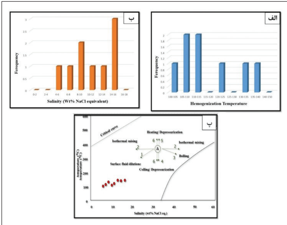
شکل ۱۲- الف) نمودار توزیع فراوانی دمای همگن شدگی در کانسار مس ساغری؛ ب) نمودار میزان شوری در میانبارهای سیال در کانسار مس ساغری (Large and et al., 1988)؛ پ) نمودار شوری در مقابل دمای همگن شدگی جهت تعیین فرایندهای مؤثر در تکامل سیال و نهشت (Wilkinson, 2001).
