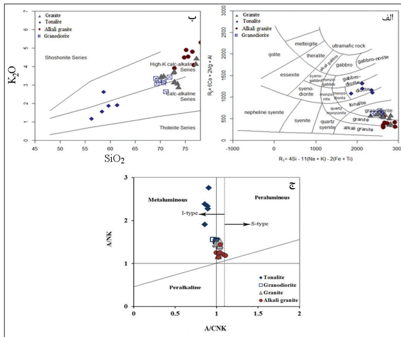
شکل ۳- الف) رده بندی سنگ های مورد مطالعه در نمودار (De La Roche et al. 1980)؛ ب) قرار گیری سنگ های مورد مطالعه در بخش سری پتاسیم تا پتاسیم بالا (Peccerillo and Taylor, 1976)؛ ج) بررسی درجه اشباع آلومینیم سنگ های مورد مطالعه (Maniar and Piccoli, 1989).
