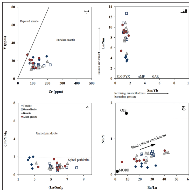
شکل ۶-الف) ترکیب کانی شناسی سنگ منشأ ماگمای مولد سنگ‌های مورد مطالعه (Kay et al., 1991)؛ ب) نمودار تفکیک ماگما باغنی شدگی بالا از ماگمای باغنی شدگی پایین (McDonough and Sun, 1988)؛ ج) نمودار Ba/La در برابر Nb/Y که تأثیر سیالات ناشی از فروانش در منشأ گرانیتوئید جبال بارز را نشان می‌دهد (داده‌های بازالت منتهی متفاوت از (Sun and McDonough 1989)؛ د) موقعیت نمونه‌های مورد مطالعه در نمودار (Wang et al., 2002).
