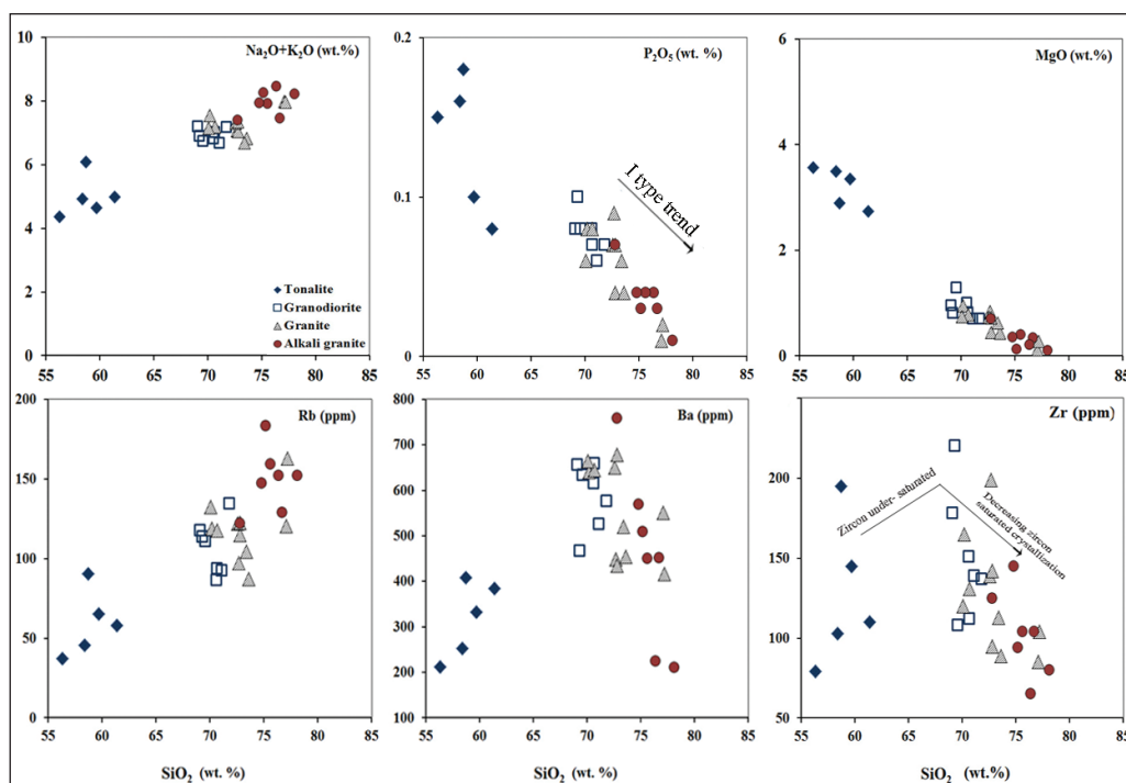
شکل ۴- نمودار تغییرات اکسید عناصر اصلی و عناصر فرعی در برابر SiO_2 .
