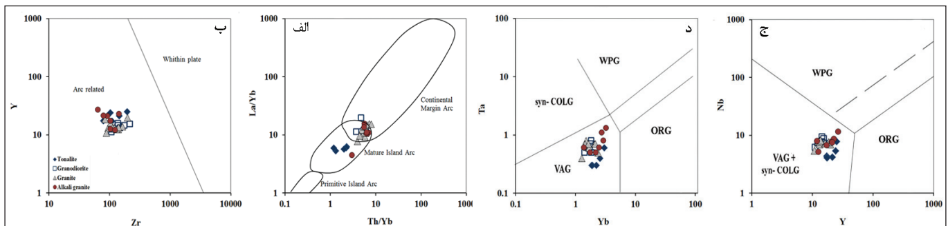
شکل ۸- موقعیت نمونه‌های مورد مطالعه: الف) در نمودار (الف) در مقابل Zr در برابر Y (Le Maitre et al., 1989)؛ ج و د) نمودارهای (Pearce et al., 1984). VAG = گرانیت‌های کمان آتشفشانی، ORG = گرانیت‌های پشته اقیانوسی و WPG = گرانیت‌های درون صفحه‌ای.
