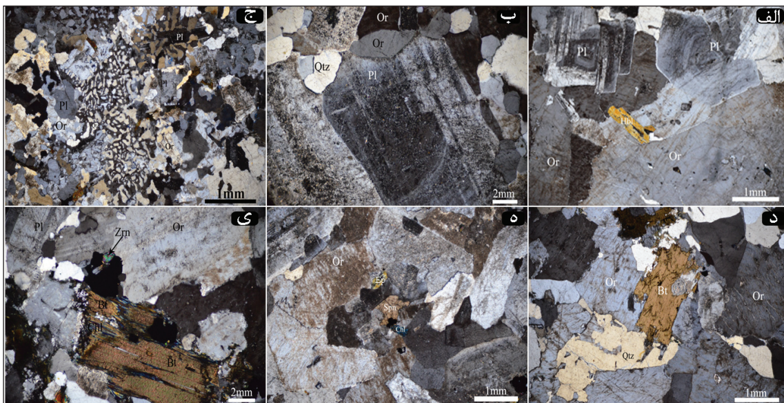
شکل ۲- نمایی از کانی‌ها و بافت‌های موجود در سنگ‌های مورد مطالعه: الف) درشت‌بلورهای پلاژیوکلاز و فلدسپار آلکالی. ب) ماکل پلی‌سنتتیک و ساختمان منطقه‌ای قابل مشاهده در پلاژیوکلازها. ج) بافت گرافیکی؛ د) بافت پرتیتی و بافت خلیجی؛ ه) اسفن اولیه؛ ی) کانی‌های کلریت و اپیدوت حاصل دگرسانی. علامت اختصاری کانی‌ها از KRBtz (1983).
