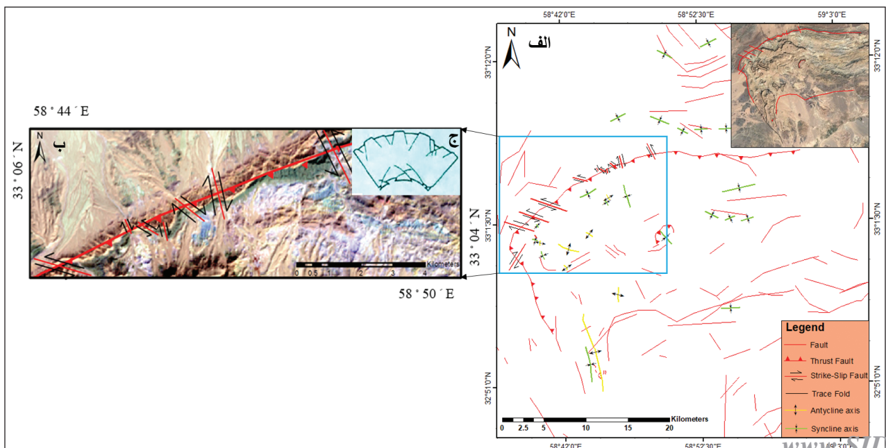
شکل ۴- الف) نقشه گسل های منطقه مطالعاتی؛ ب) نمایی از گسل های برشی مزدوج در پیشانی قوس بر روی تصاویر ماهواره ای؛ ج) نمایش الگوی چین خوردگی از نوع Buckling.
