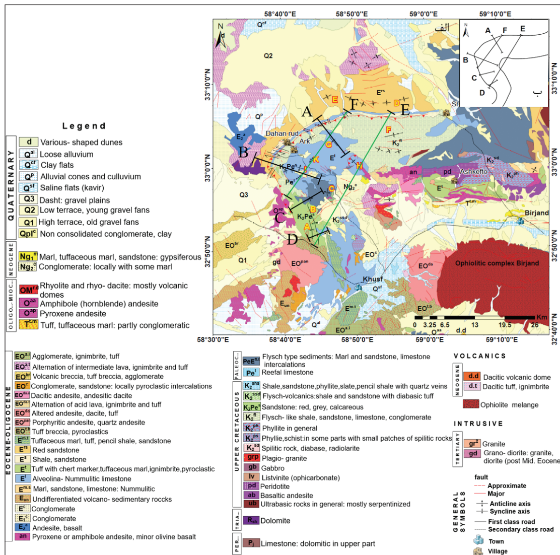
شکل ۲ الف) نقشه زمین‌شناسی ساده‌شده از قوس ساختاری شمال غرب بیرجند برگرفته از نقشه‌های زمین‌شناسی بیرجند و قائن (Berthiaux et al., 1991). ب) نمایش شماتیک برش‌های زمین‌شناسی. (Vahdati Daneshmand et al., 1991) که حروف زرد رنگ در آن چین‌های شعاعی و موازی را نشان می‌دهد؛
